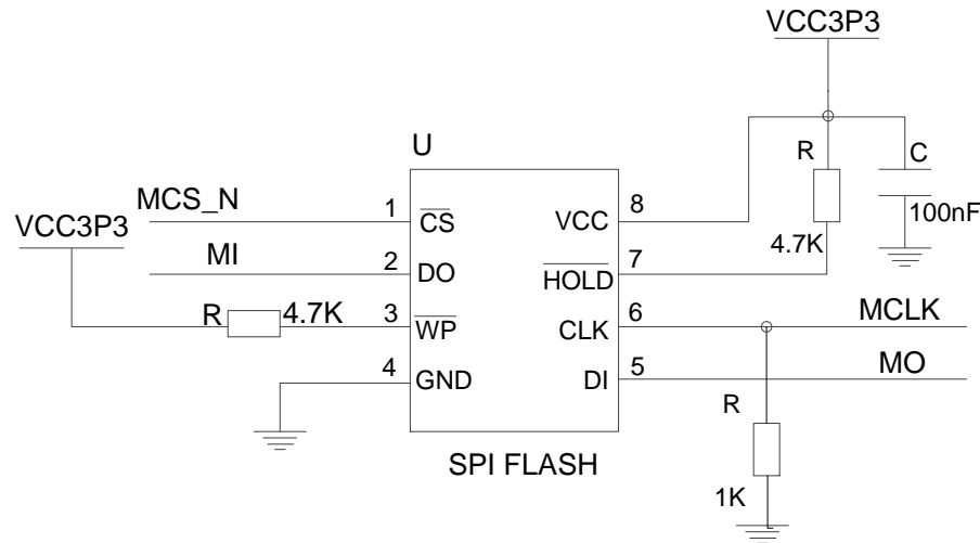
图 4 MSPI 电路参考
