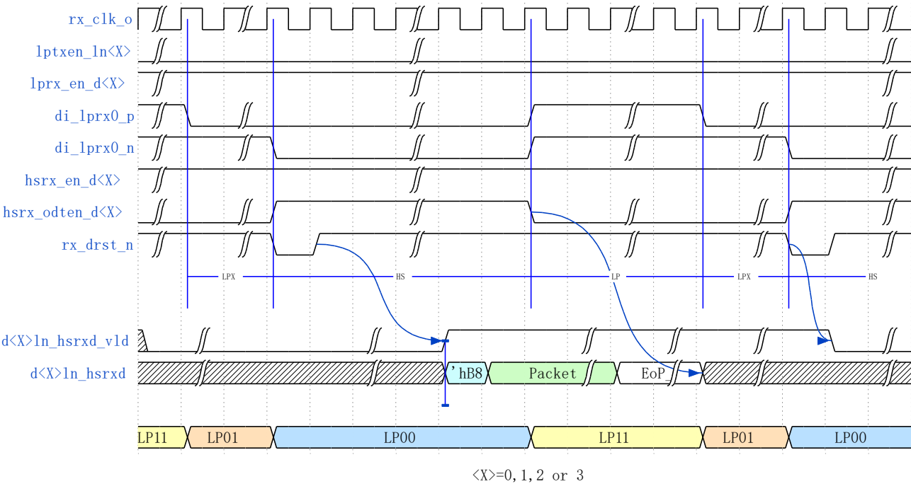
图 4-3 MIPI D-PHY RX 典型时序
