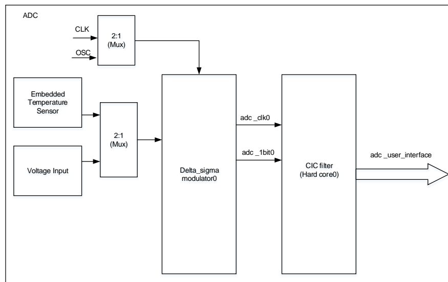
图 2-1 25K 器件 ADC 结构框图
