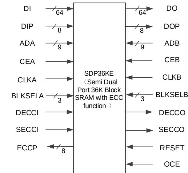
图 3-12 SDP36KE 端口示意图
