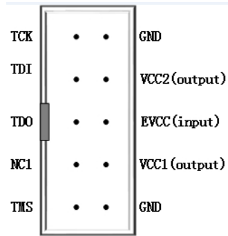
图 2-14 烧录接口连线示意图
