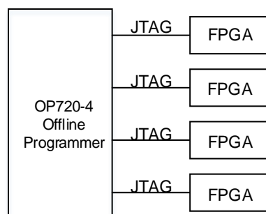
图 2-12 烧录器与 SocketBoard 连接示意图
