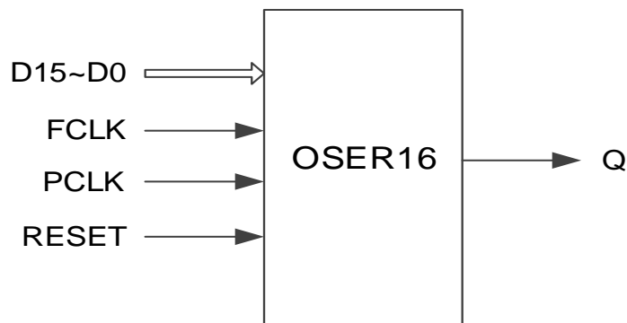
图 4-37 OSER16 端口示意图
