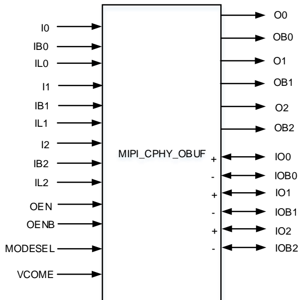
图 3-16 MIPI_CPHY_OBUF 端口示意图
