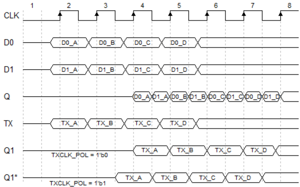
图 4-27 ODDR 时序图
