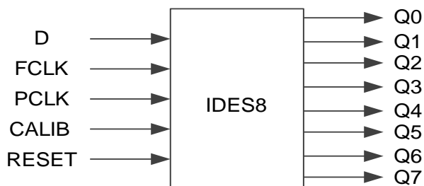
图 4-15 IDES8 端口示意图
