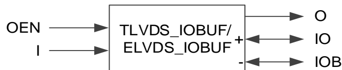
图 3-12 TLVDS_IOBUF/ELVDS_IOBUF 端口示意图
