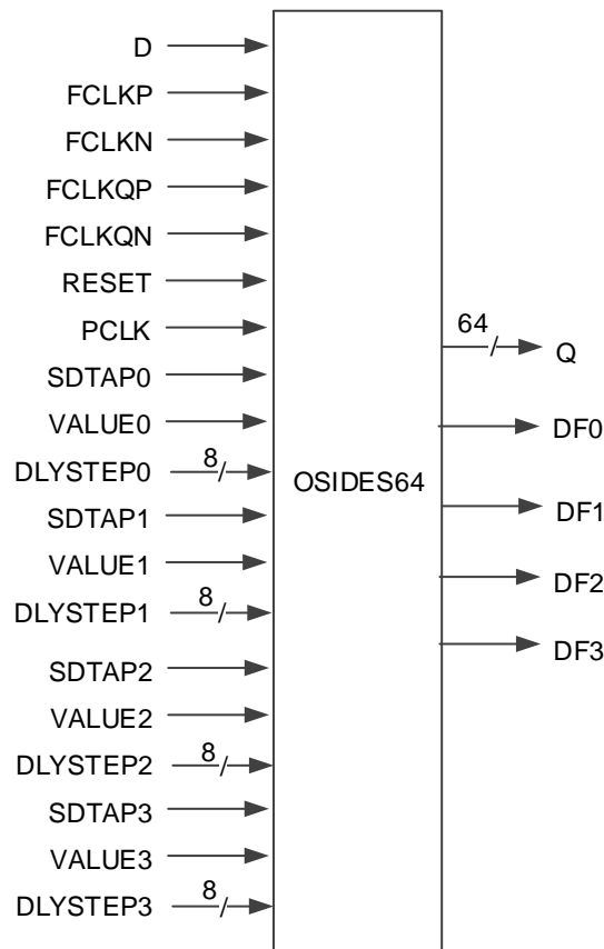
图 4-25 OSIDES64 端口示意图
