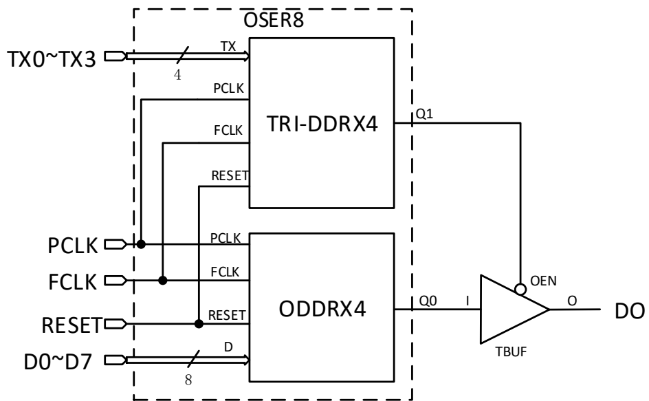
图 4-33 OSER8 逻辑框图
