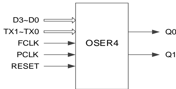
图 4-32 OSER4 端口示意图
