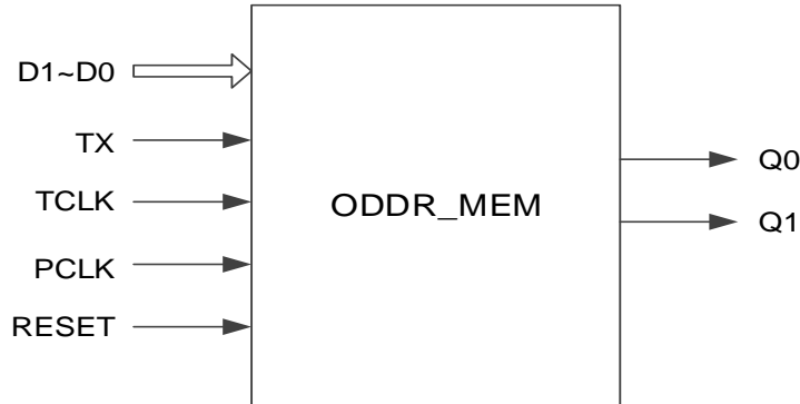
图 4-39 ODDR_MEM 端口示意图
