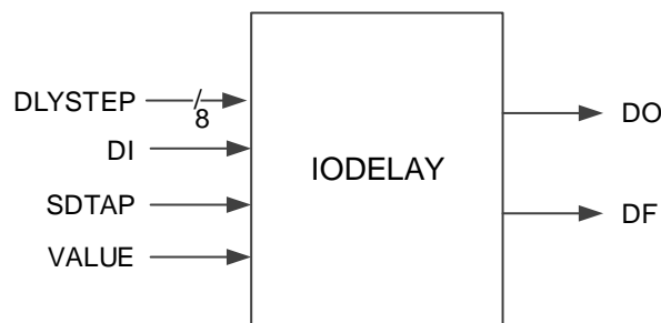
图 4-44 IODELAY 端口示意图
