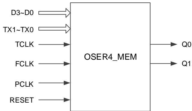
图 4-41 OSER4_MEM 端口示意图
