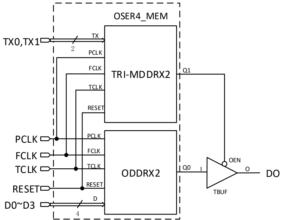
图 4-40 OSER4_MEM 逻辑框图
