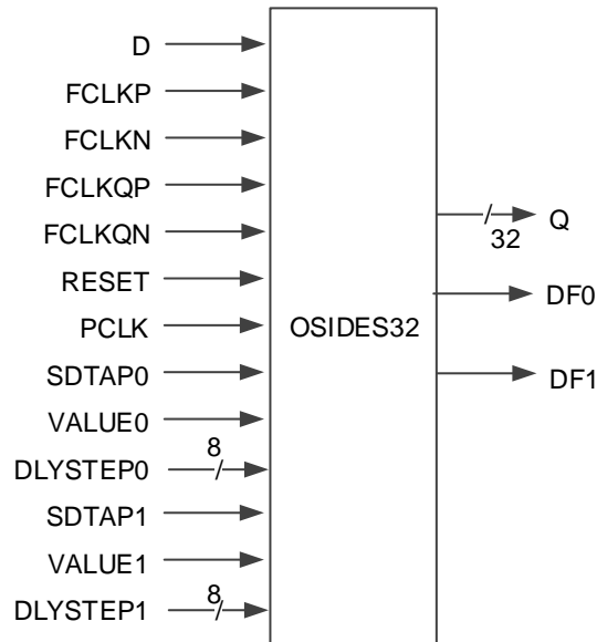
图 4-24 OSIDES32 端口示意图
