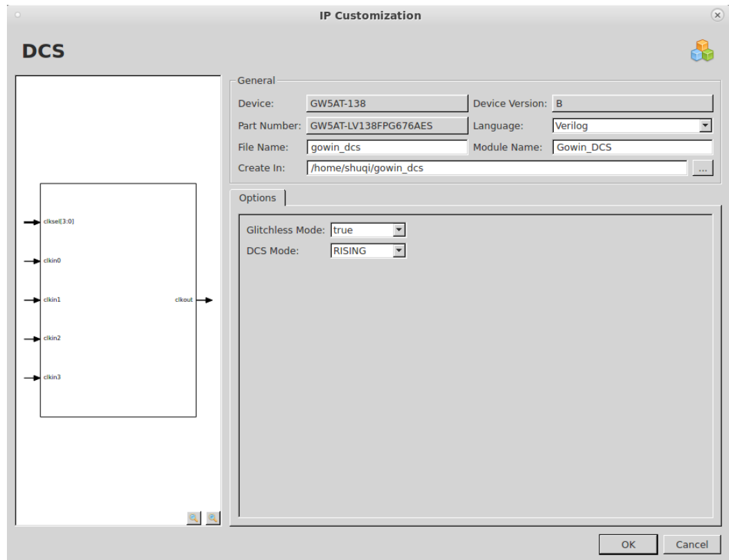
图 3-9 DCS 的 IP Customization 窗口结构
