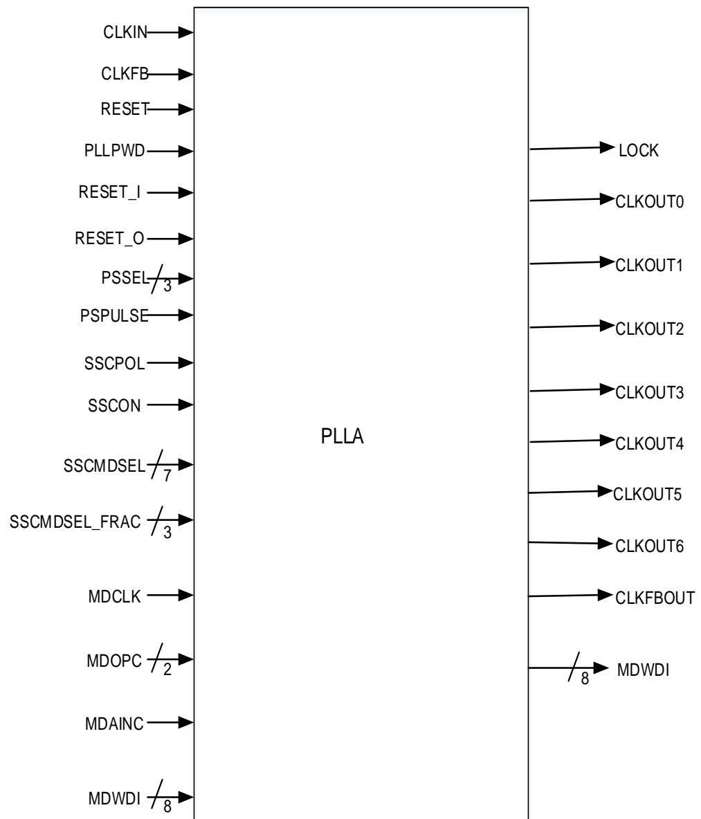
图 5-7 PLLA 端口示意图
