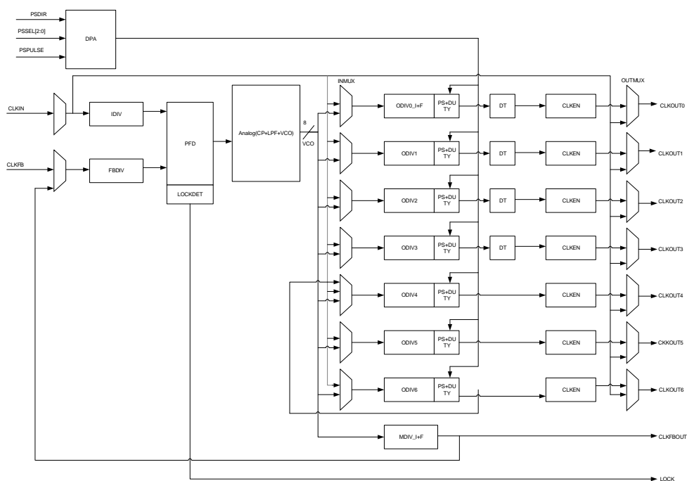
图 5-6 PLLA 示意图
