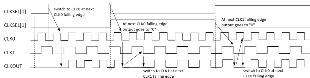
图 3-6 DCS mode: FALLING 时序图
