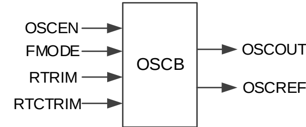
图 6-5 OSCB 端口示意图
