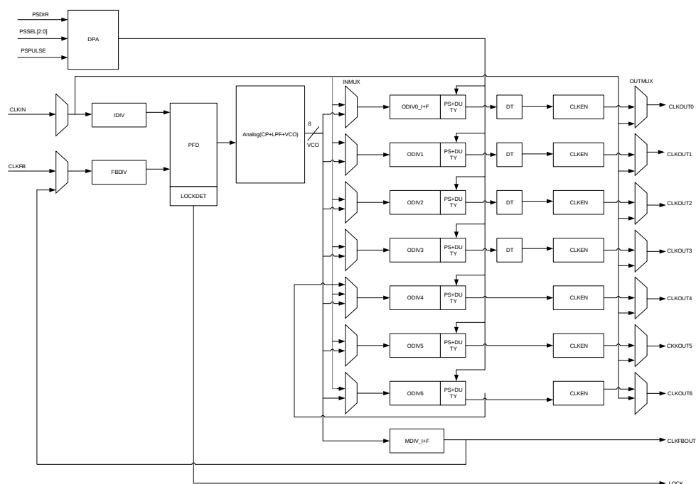
图 5-1 PLL 示意图
