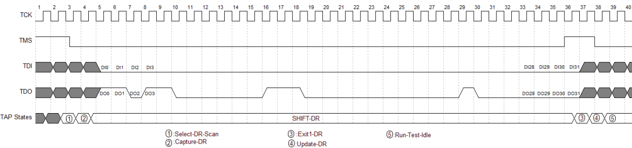
图 3-11 读取 ID Code 数据寄存器访问时序
