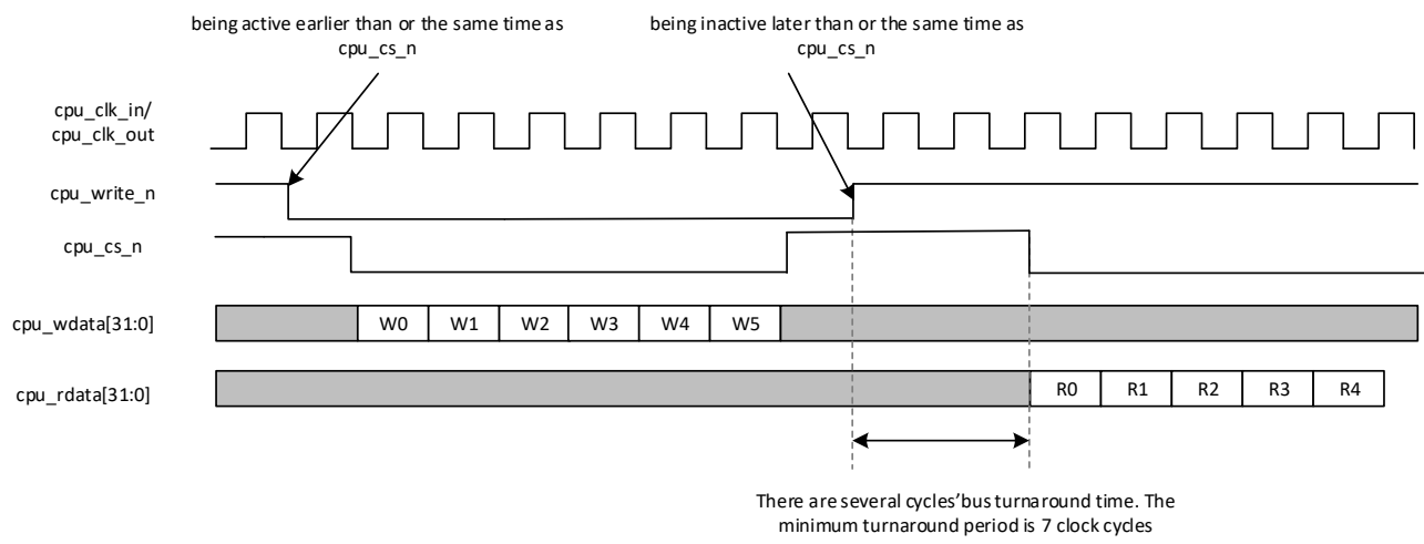
图 3-37 连续加载时序图
