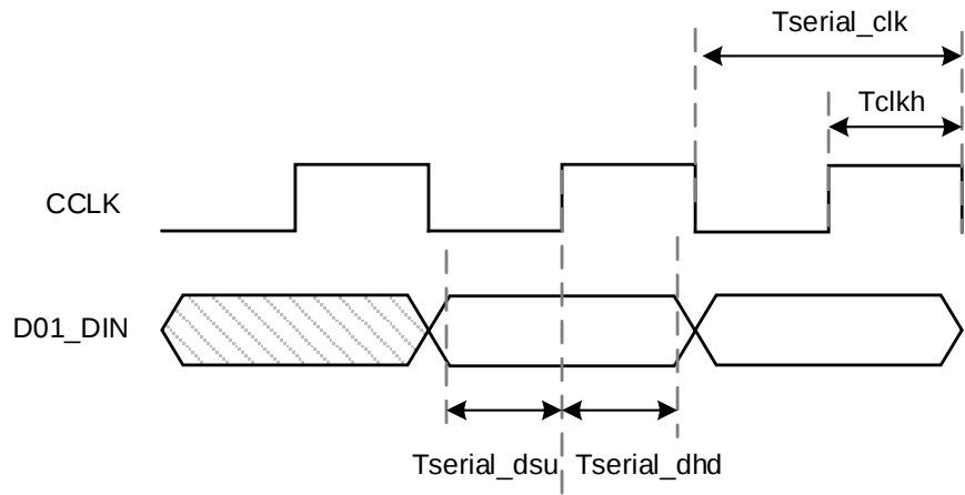
图 3-40 SERIAL 配置模式时序图
