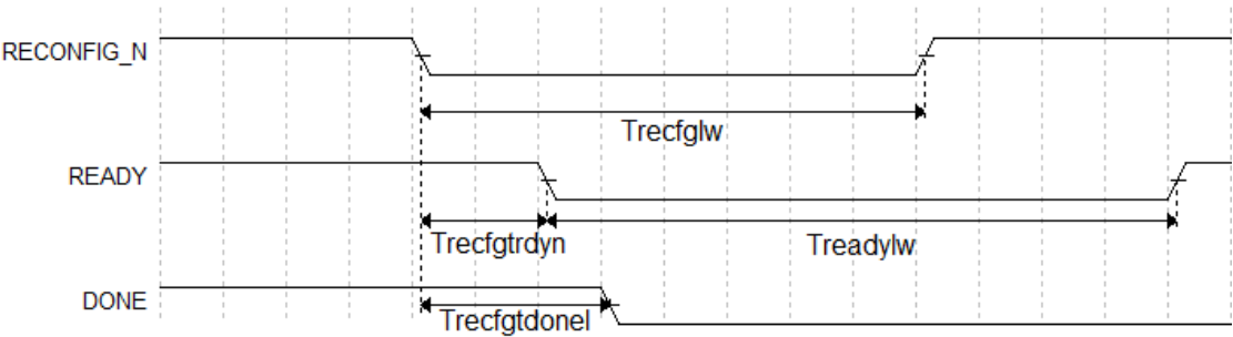
图 4-3 触发时序图
