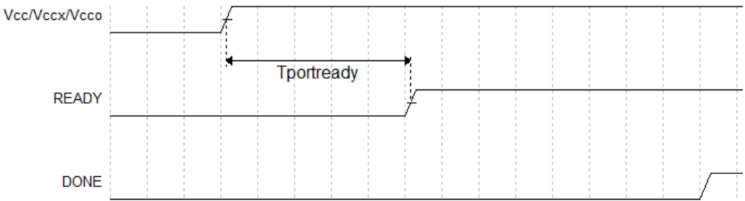
图 4-3 触发时序图
