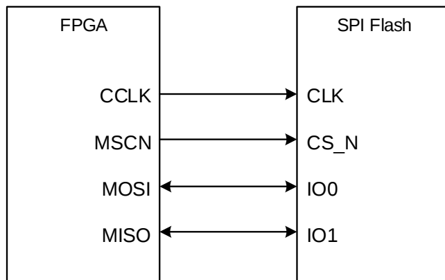
图 3-31 MSPIx2 配置模式连接示意图
