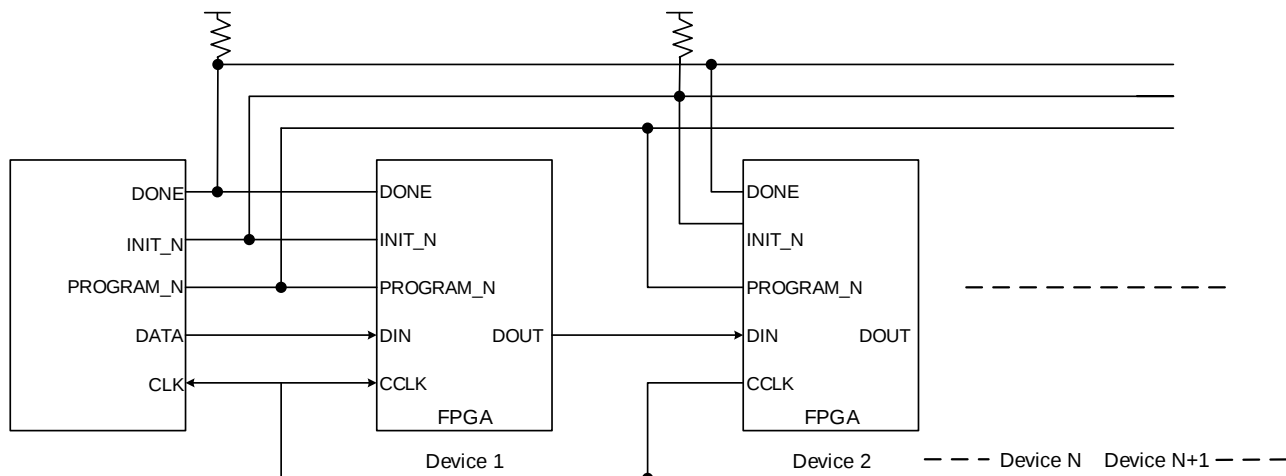
图 3-41 串行菊花链示意图
