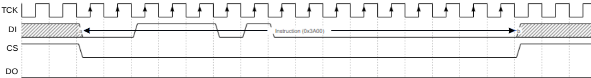
图 3-24 Write Disable (0x3A00) 时序示意图
