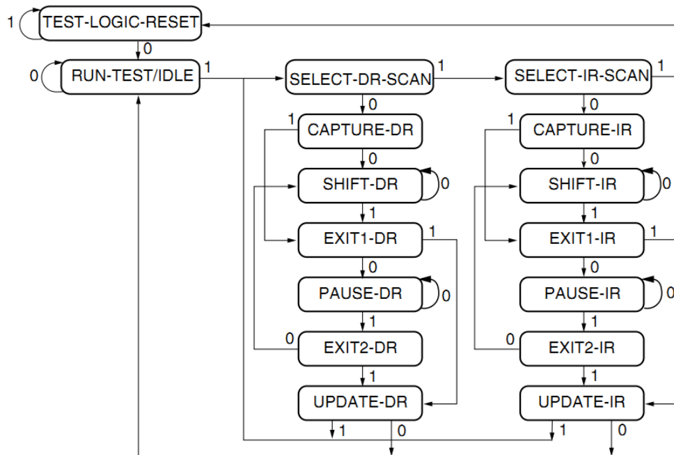
图 3-6 TAP 状态机
