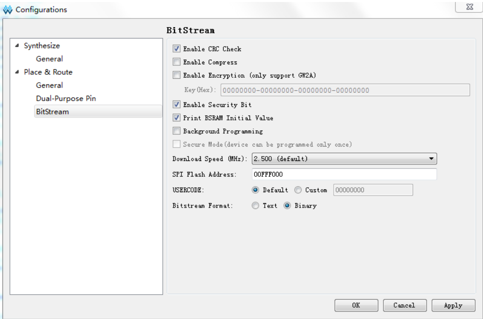
图 4-15 比特流格式生成
