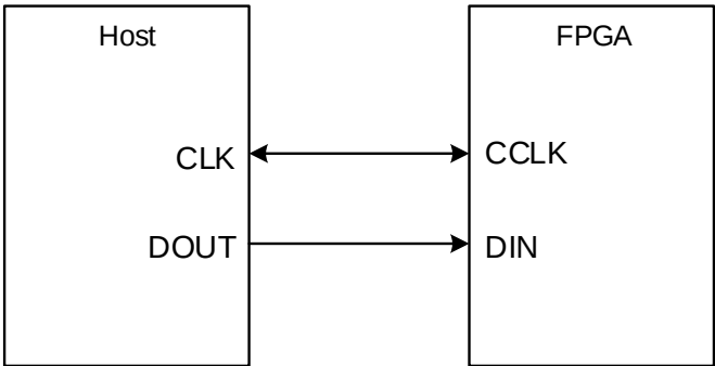
图 3-39 SERIAL 配置模式连接示意图
