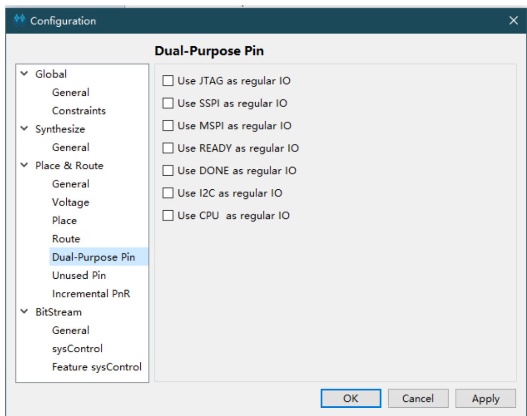
图 3-1 配置管脚复用设置
