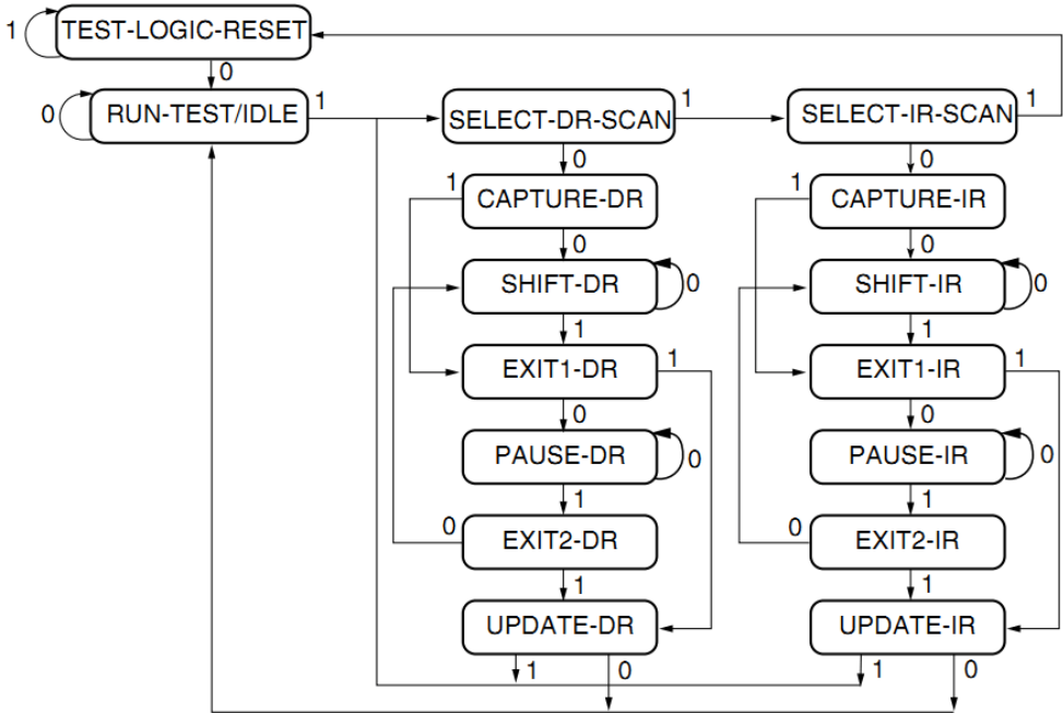
图 3-6 TAP 状态机
