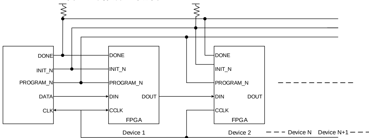
图 3-41 串行菊花链示意图
