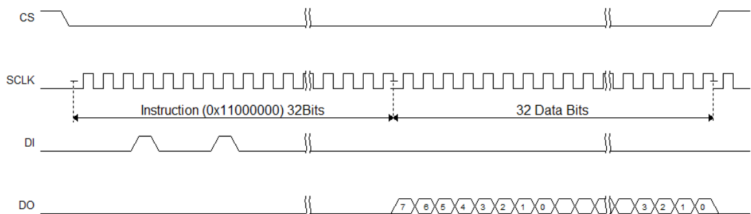
图 3-23 读取 ID Code 时序示意图
