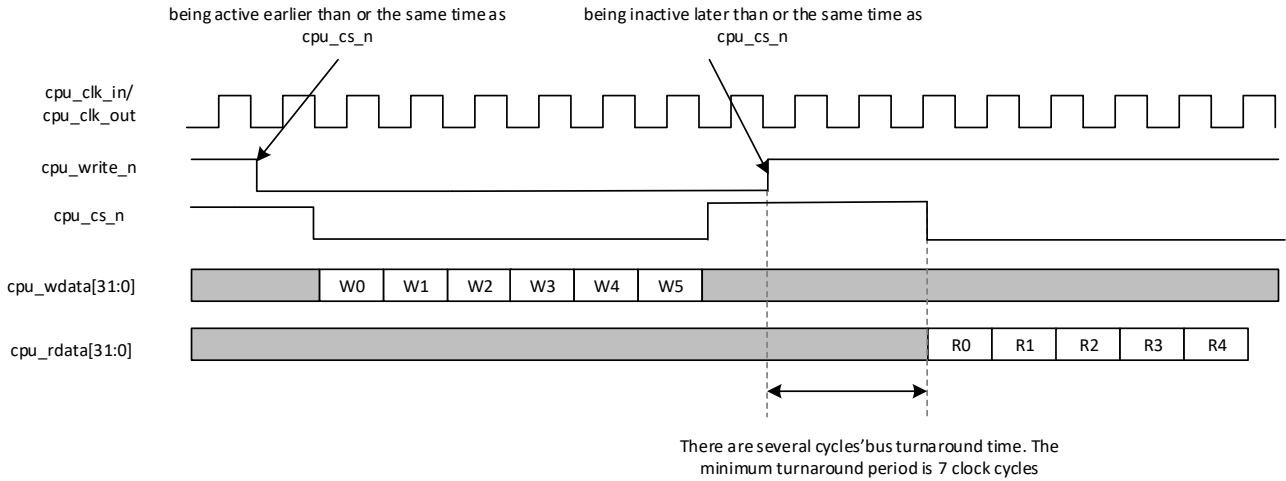
图 3-39 连续加载时序图
