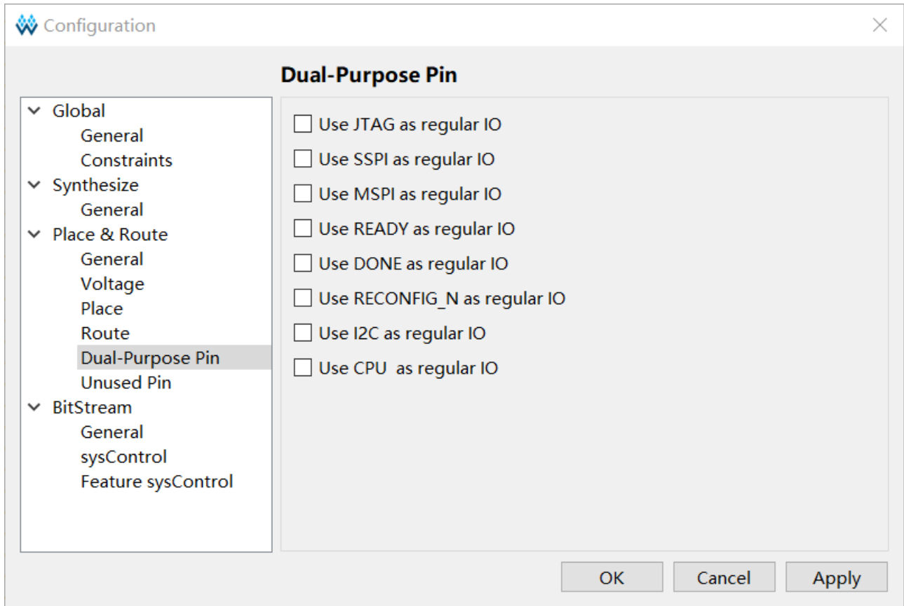
图 3-1 配置管脚复用设置
