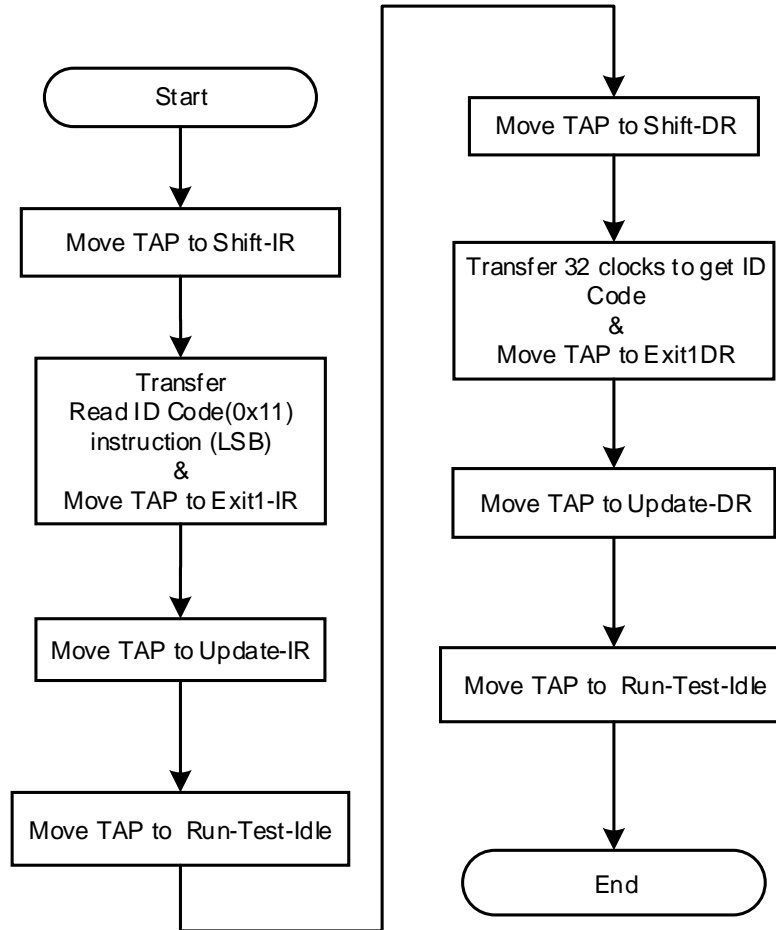
图 3-10 读取 ID Code 指令-0x11 访问时序
