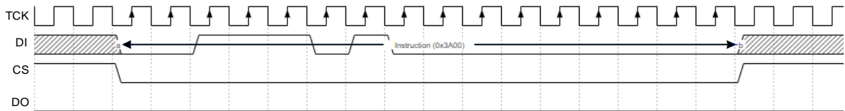
图 3-25 Write Disable (0x3A00) 时序示意图
