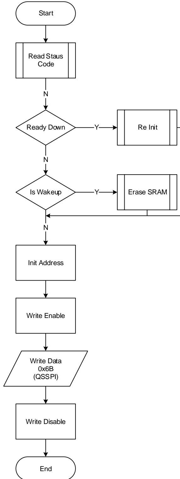
图 3-29 QSSPI 配置 SRAM 流程图
