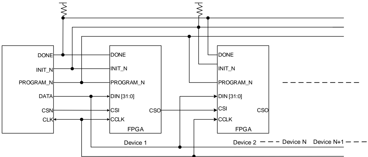
图 3-44 并行菊花链示意图
