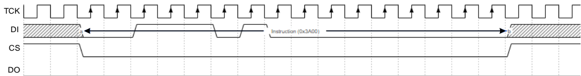
图 3-24 Write Disable (0x3A00) 时序示意图
