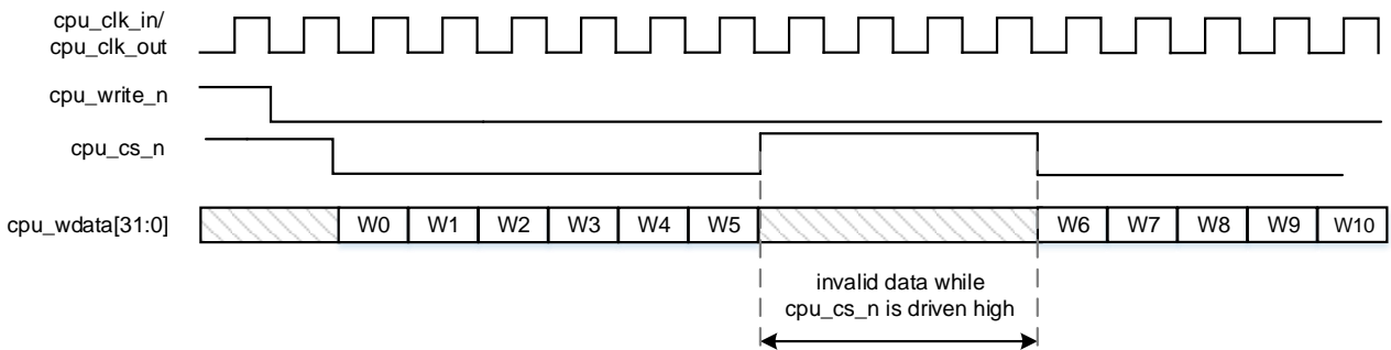
图 3-39 非连续加载时序图
