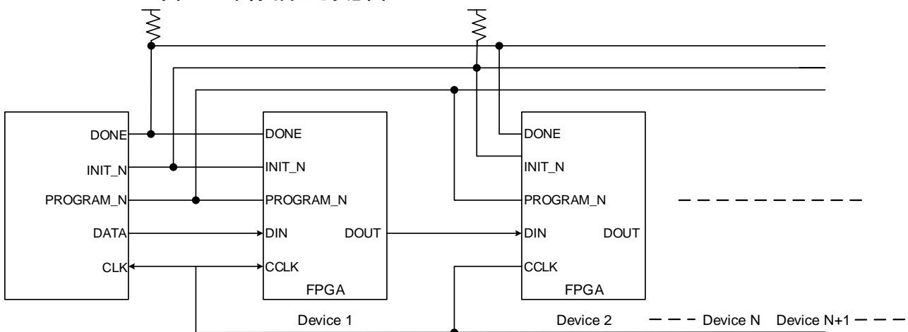
图 3-42 串行菊花链示意图
