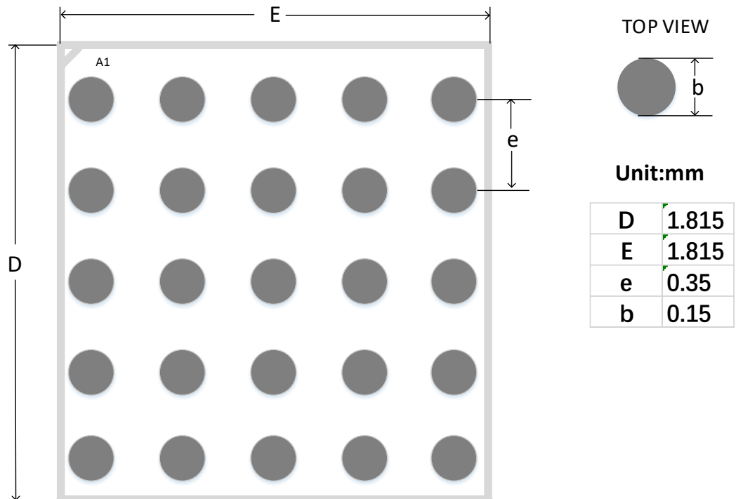
图 4-12 推荐 PCB Layout CG25
