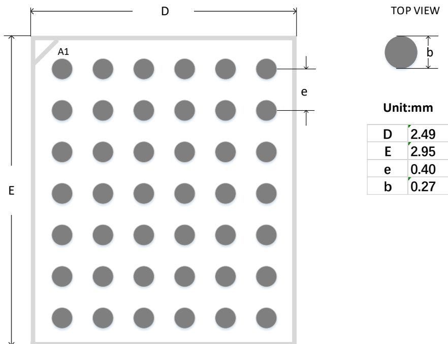
图 4-16 推荐 PCB Layout CS42
