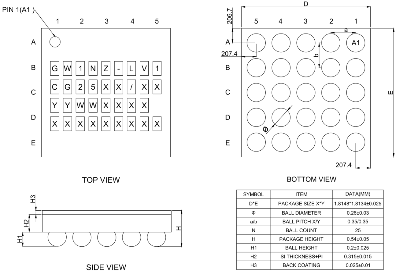
图 4-11 封装尺寸 CG25
