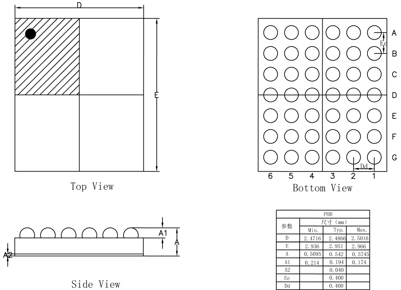
图 4-15 封装尺寸 CS42
