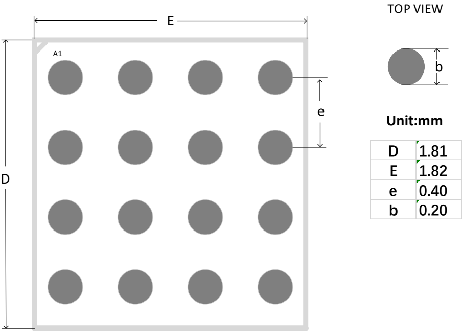
图 4-4 推荐 PCB Layout CS16
