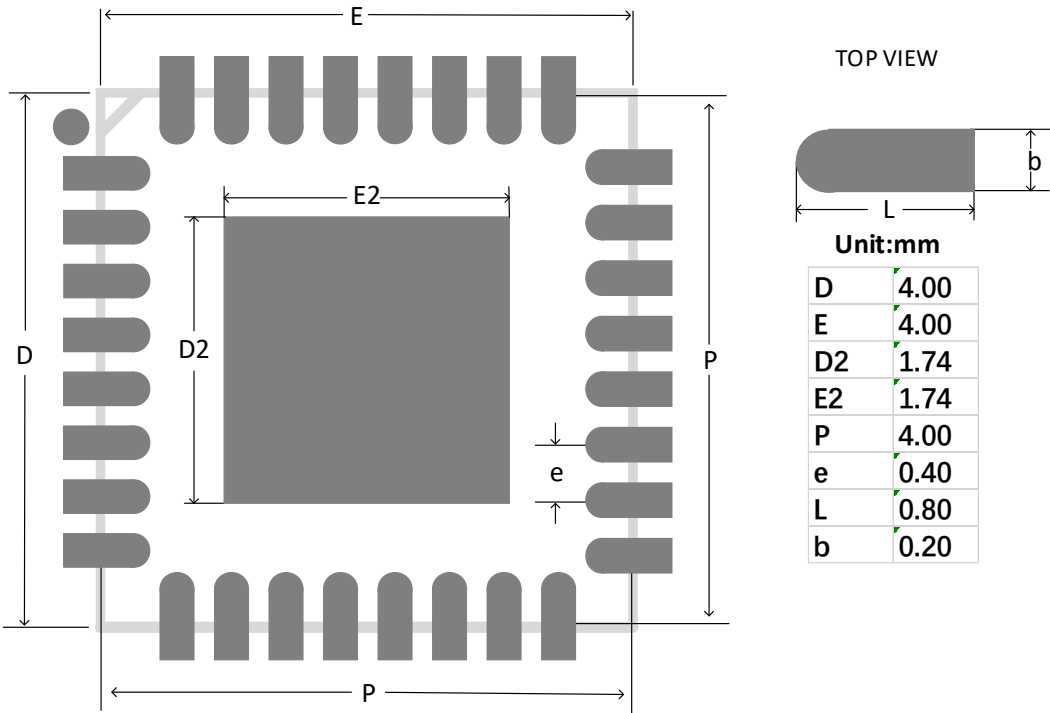
图 4-16 推荐 PCB Layout FN32F
