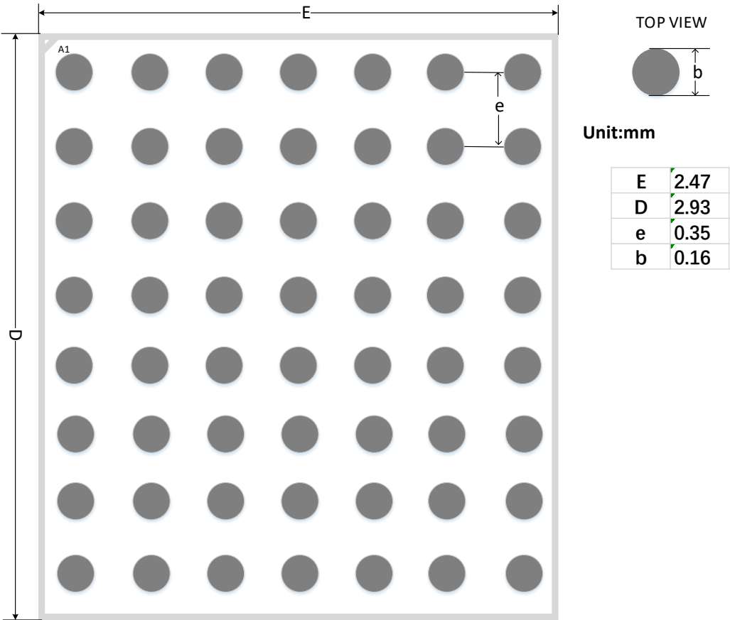
图 4-10 推荐 PCB Layout CG56
