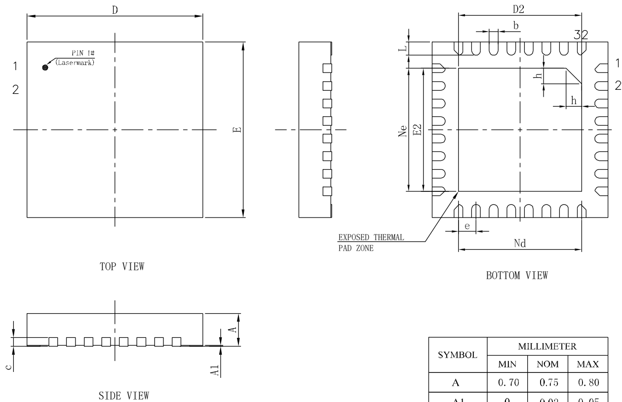
图 4-13 封装尺寸 FN32
