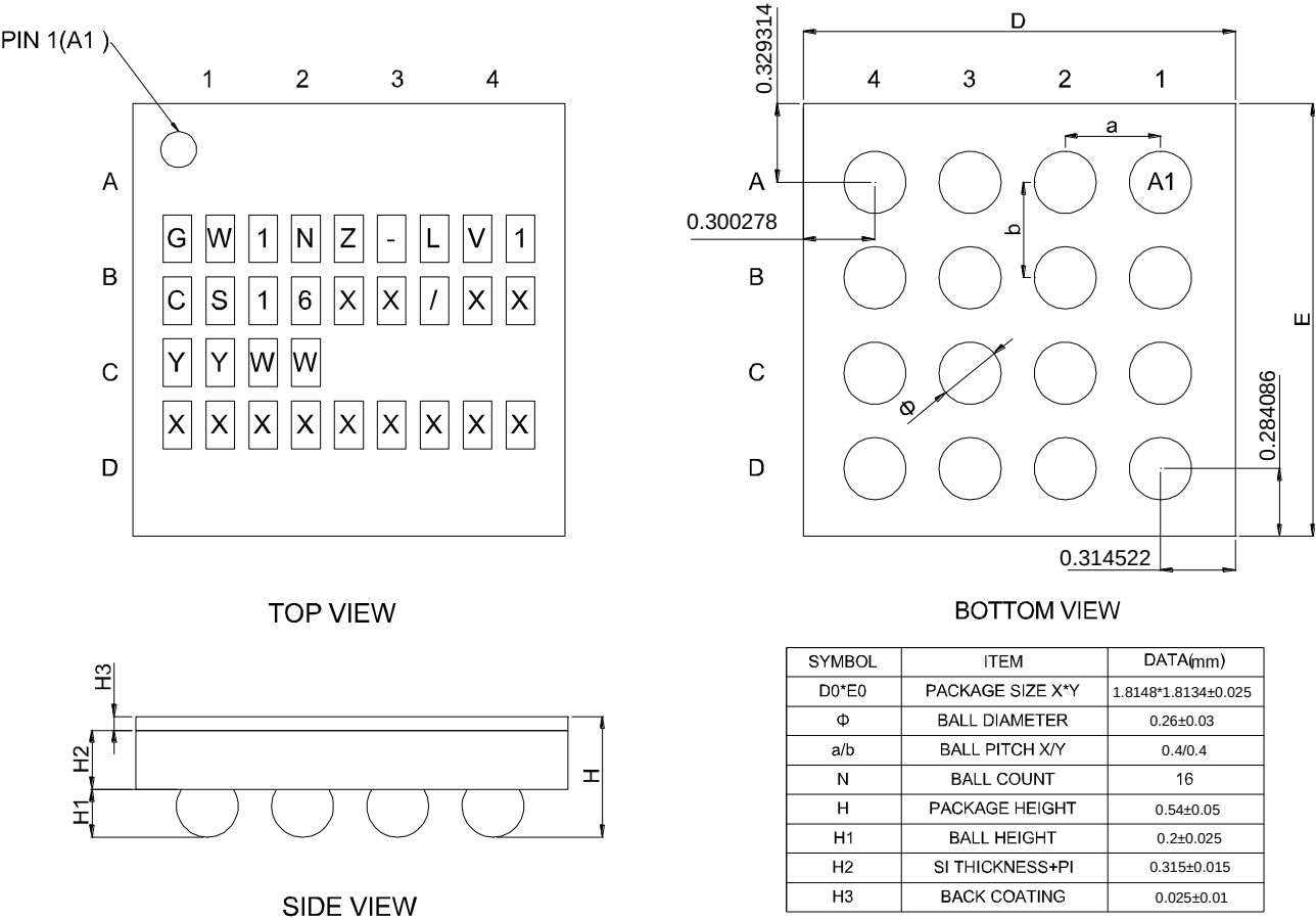
图 4-3 封装尺寸 CS16
