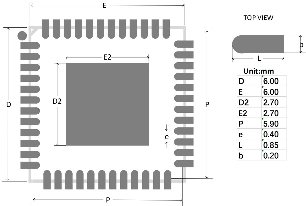
图 4-18 推荐 PCB Layout QN48
