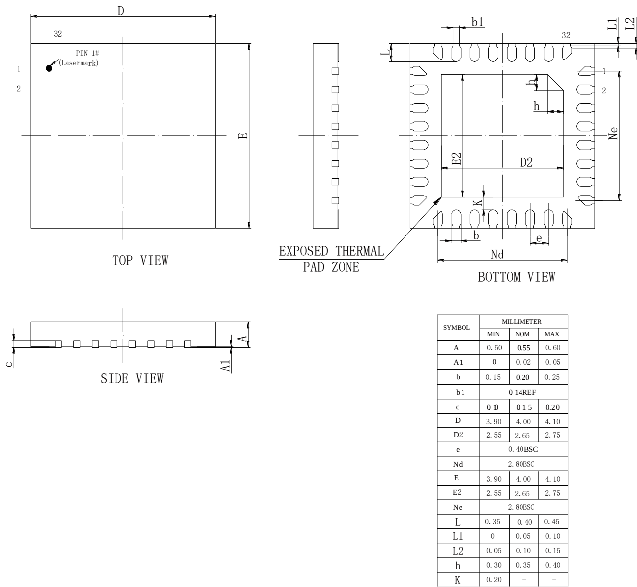
图 4-15 封装尺寸 FN32F
