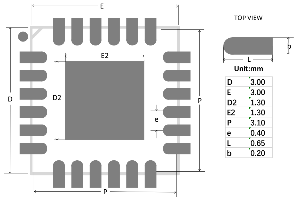
图 4-12 推荐 PCB Layout FN24
