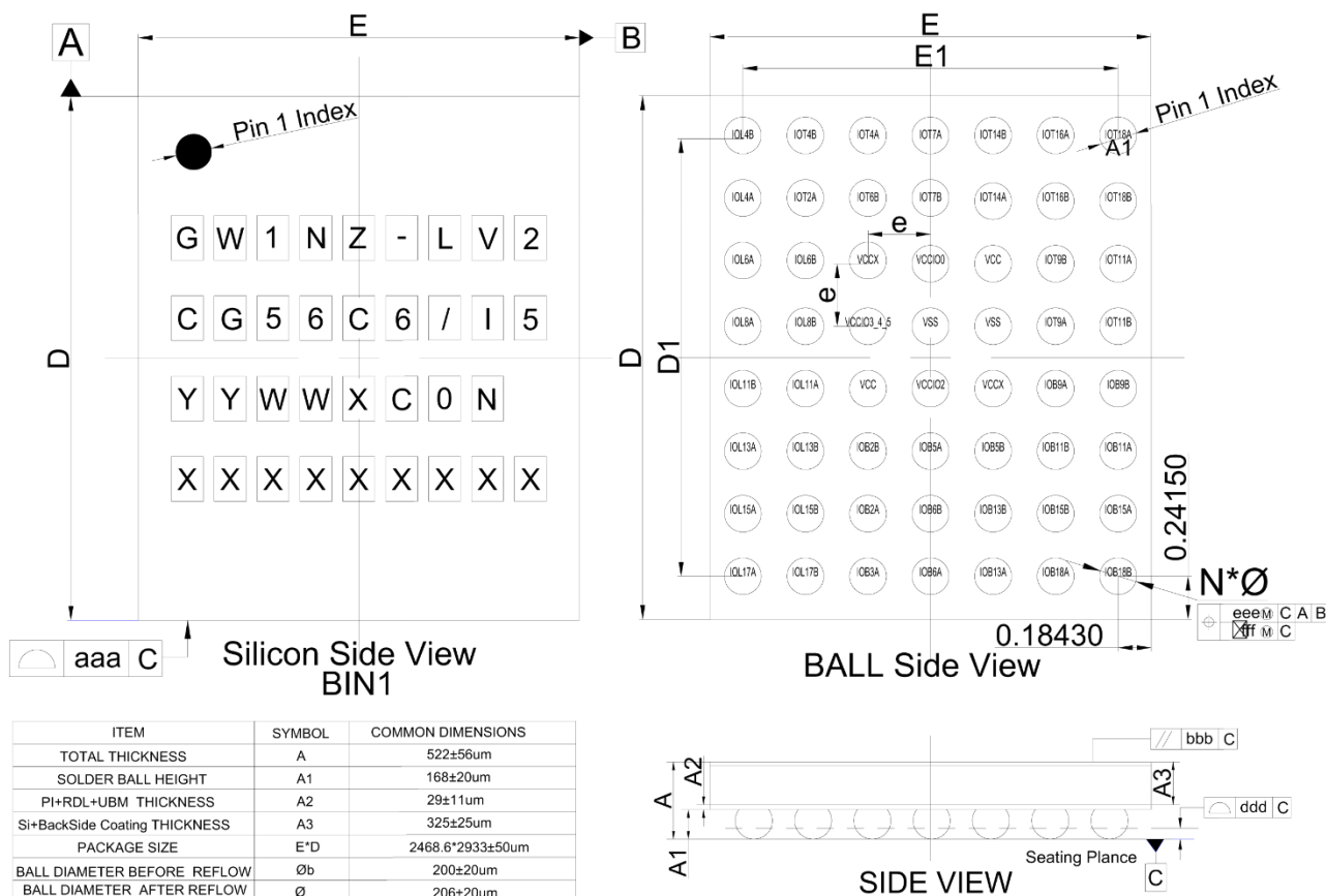
图 4-9 封装尺寸 CG56
