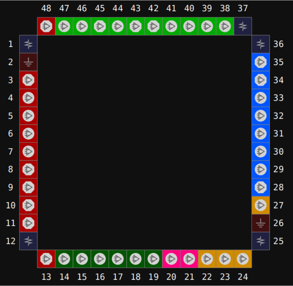
图 3-10 GW1NZ-2 器件 QN48 封装管脚分布示意图（顶视图）
