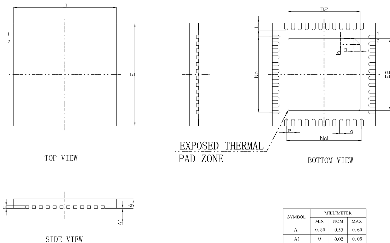
图 4-17 封装尺寸 QN48
