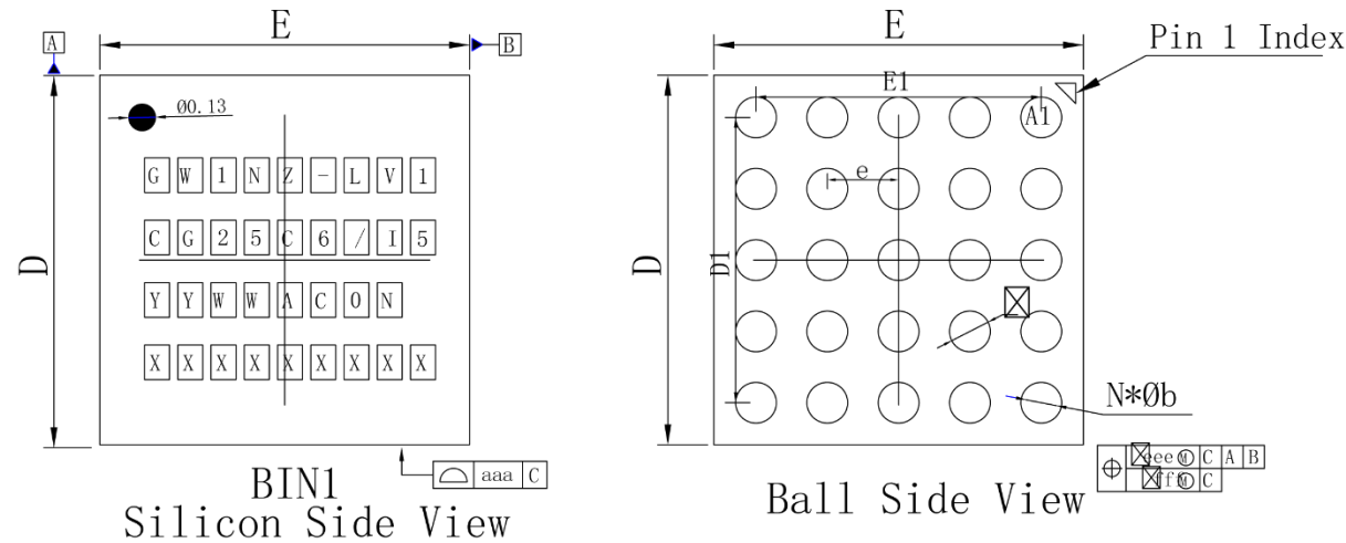
图 4-5 封装尺寸 CG25
