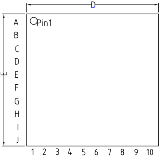
图 4-1 封装尺寸 CS100H
