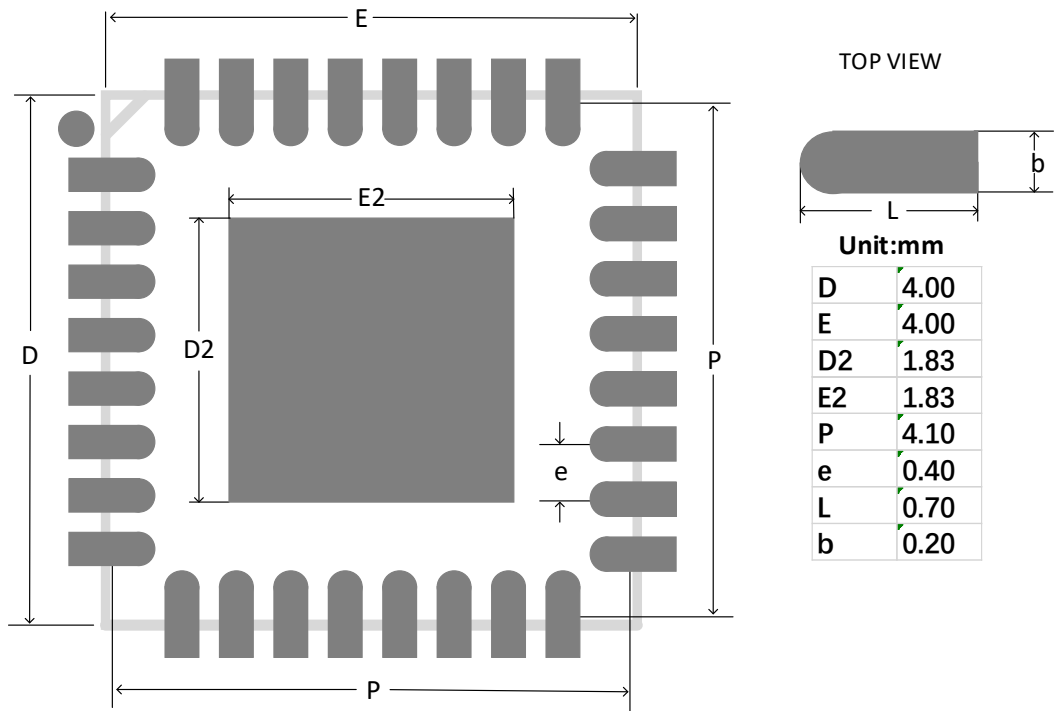
图 4-14 推荐 PCB Layout FN32
