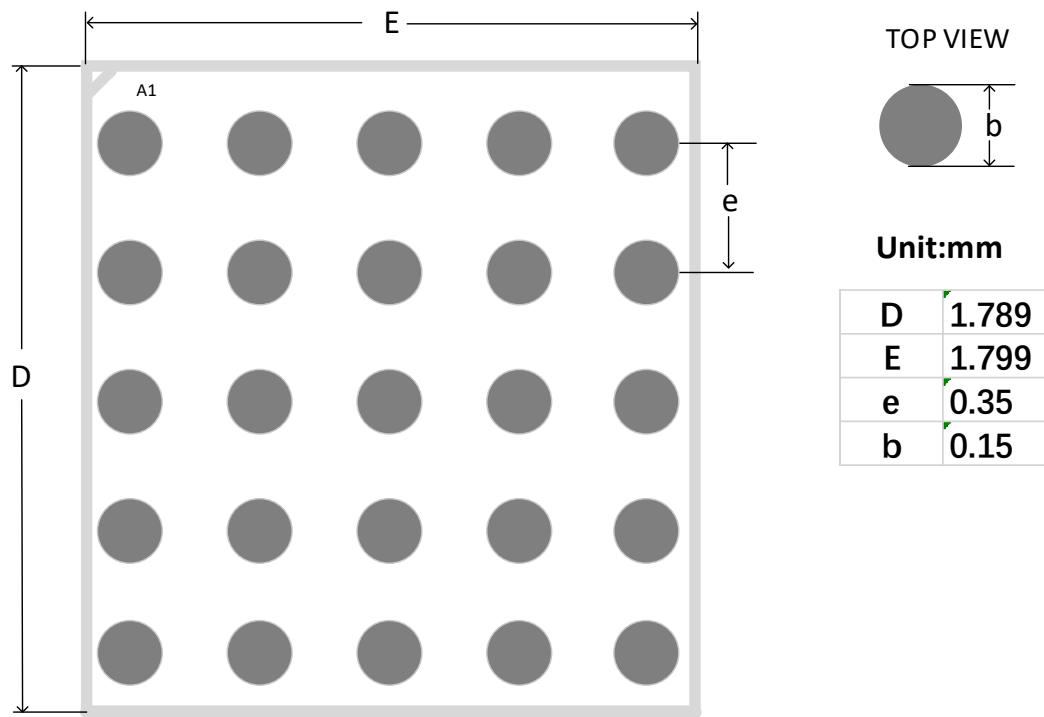
图 4-6 推荐 PCB Layout CG25
