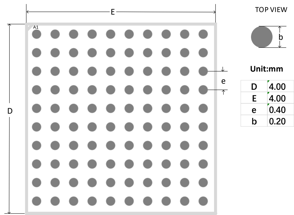
图 4-2 推荐 PCB Layout CS100H
