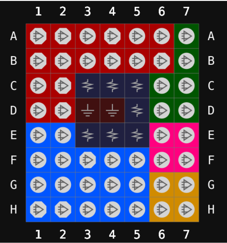
图 3-9 GW1NZ-2 器件 CG56 封装管脚分布示意图（顶视图）
