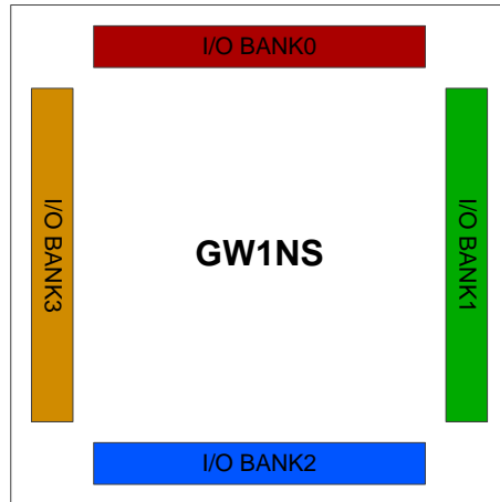
图 2-1 GW1NSER 系列安全 FPGA 产品 I/O BANK 整体示意图
