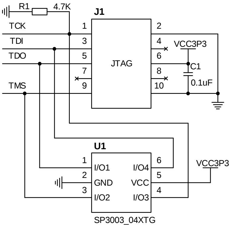
图 3 JTAG 电路
