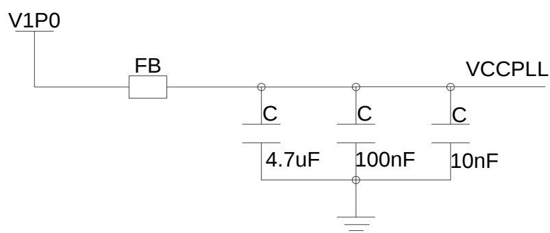
图 2 隔离滤波 V CCPLL
