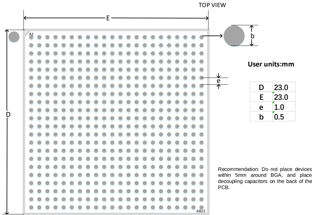
图 4-4 推荐 PCB Layout PG484A
