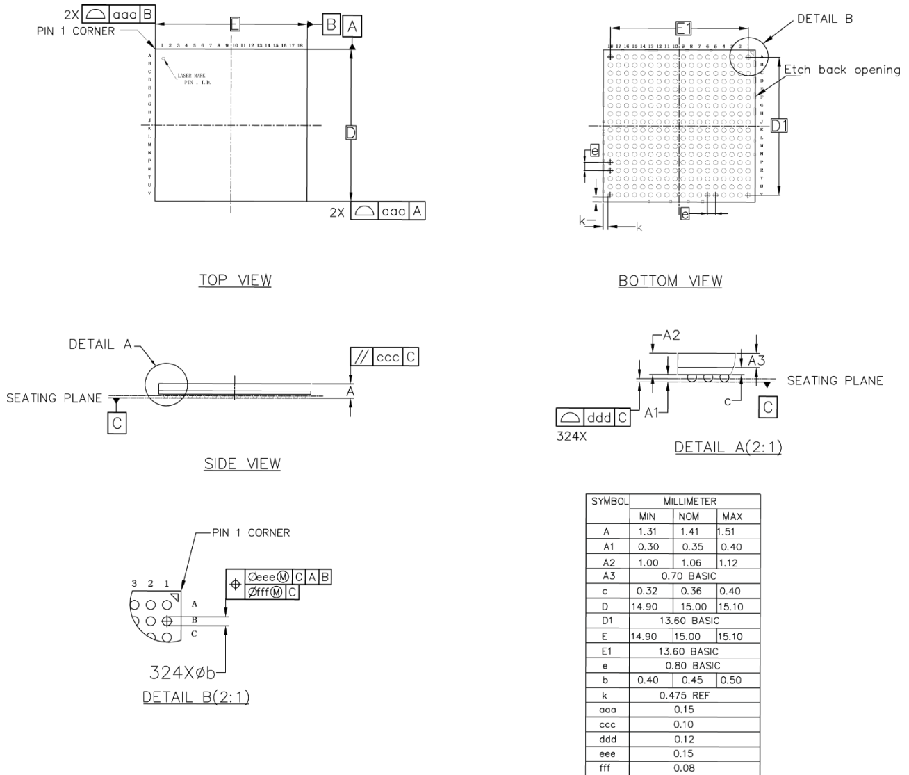
图 4-11 封装尺寸 UG324A
