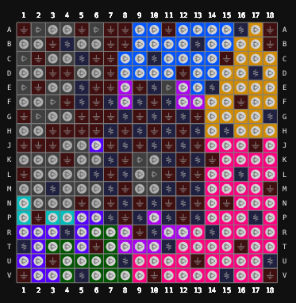
图 3-5 GW5AT-138 器件 UG324 封装管脚分布示意图（顶视图）
