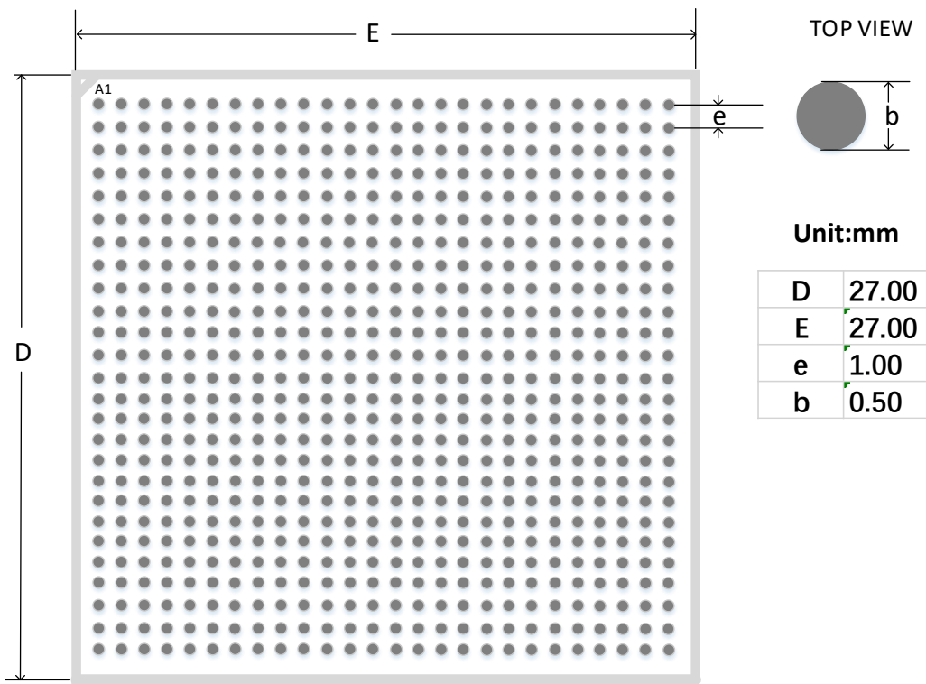
图 4-8 推荐 PCB Layout PG676A
