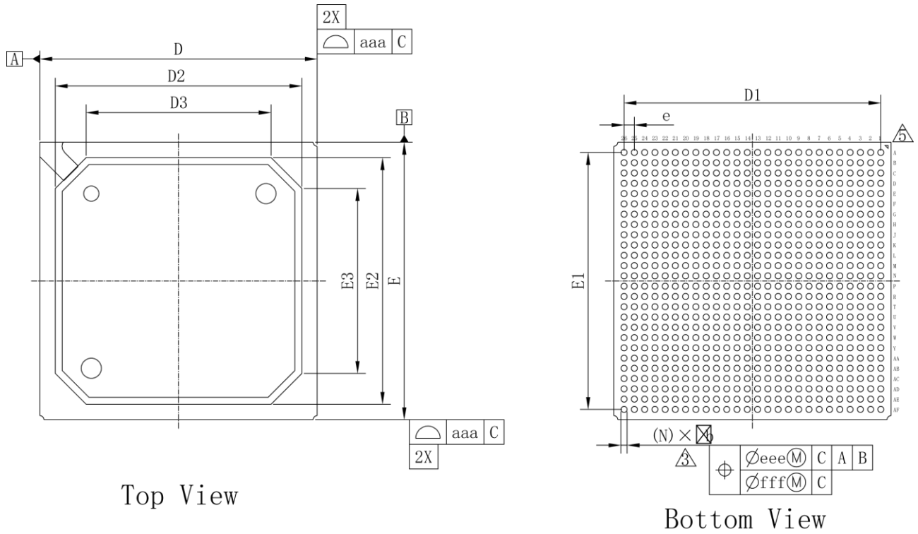
图 4-7 封装尺寸 PG676A
