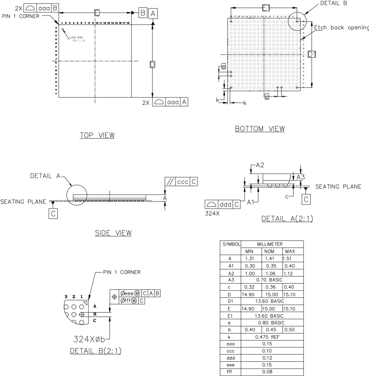
图 4-9 封装尺寸 UG324
