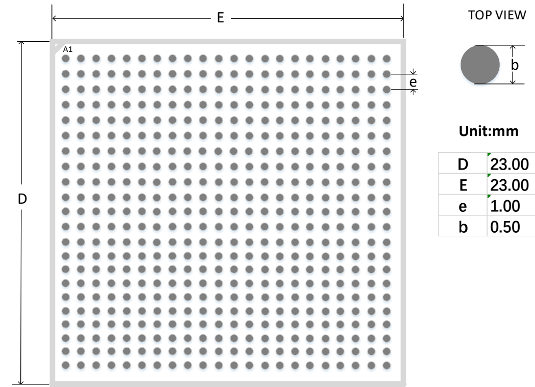
图 4-6 推荐 PCB Layout PG484
