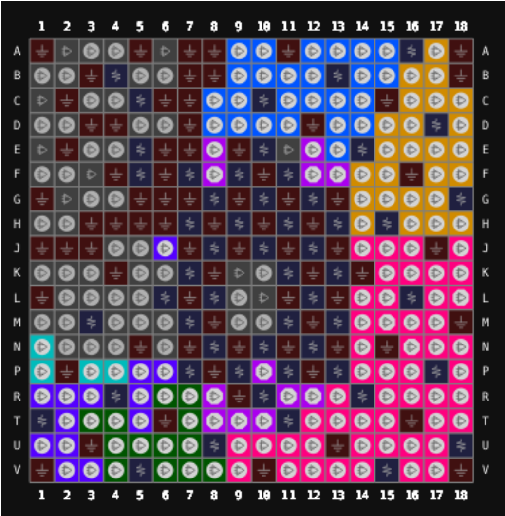
图 3-6 GW5AT-138 器件 UG324A 封装管脚分布示意图（顶视图）
