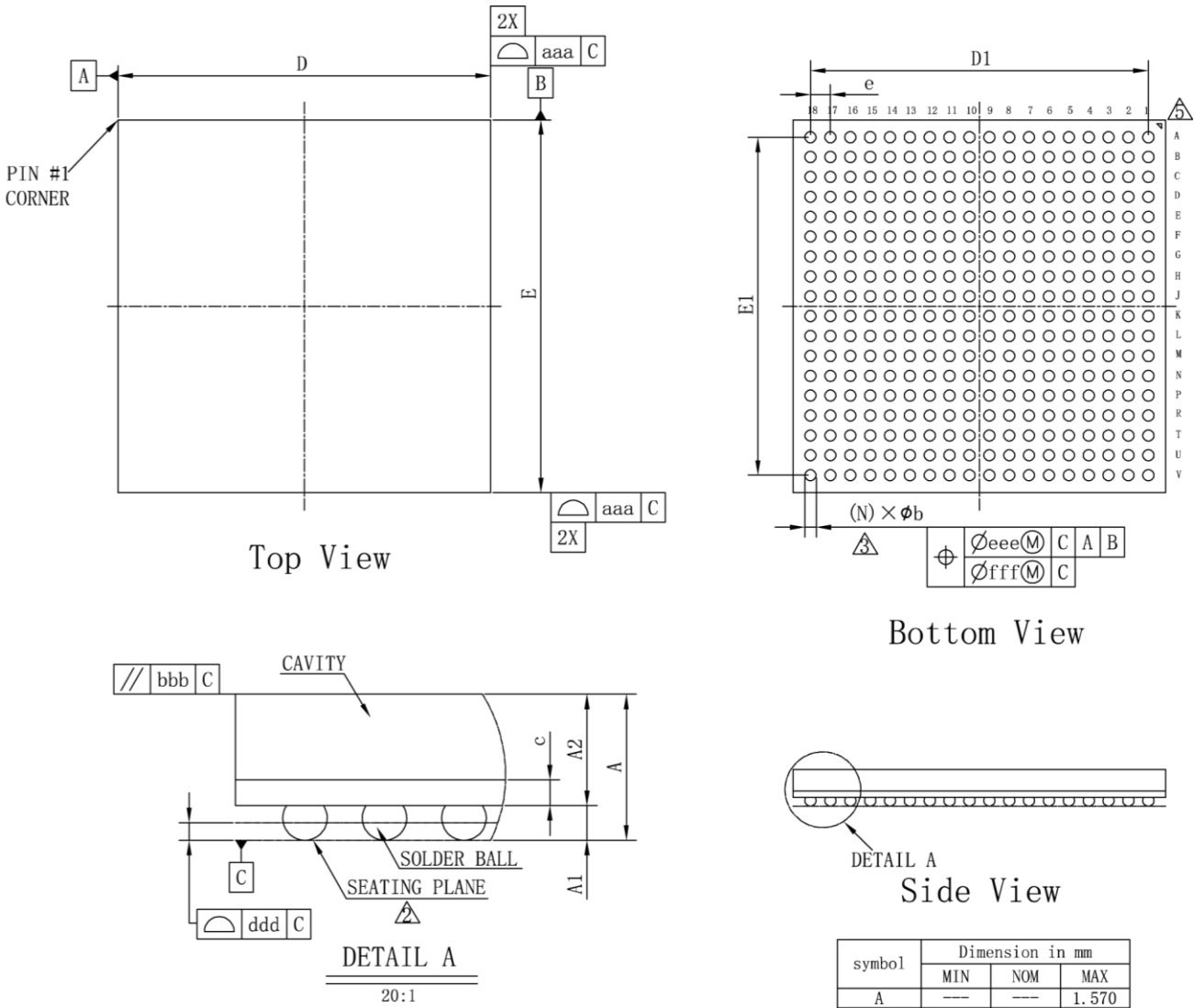
图 4-23 封装尺寸 UG324 (GW5AT-60)
