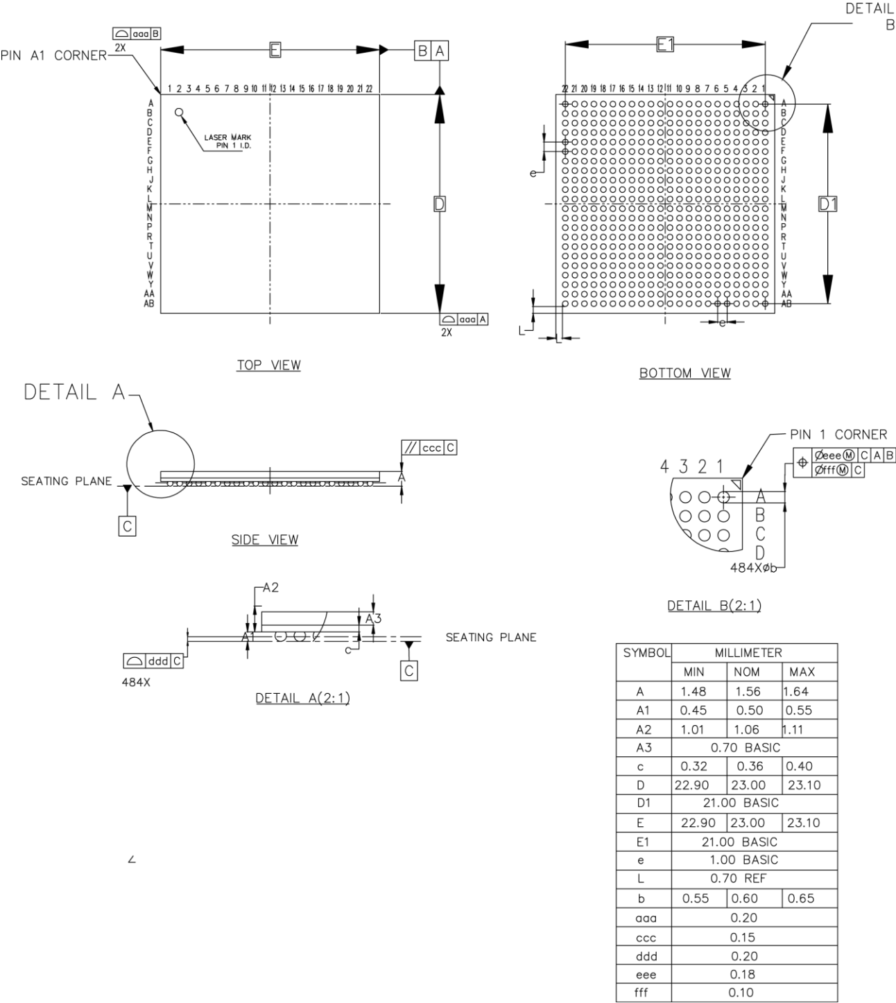
图 4-13 封装尺寸 PG484A (GW5AT-138)
