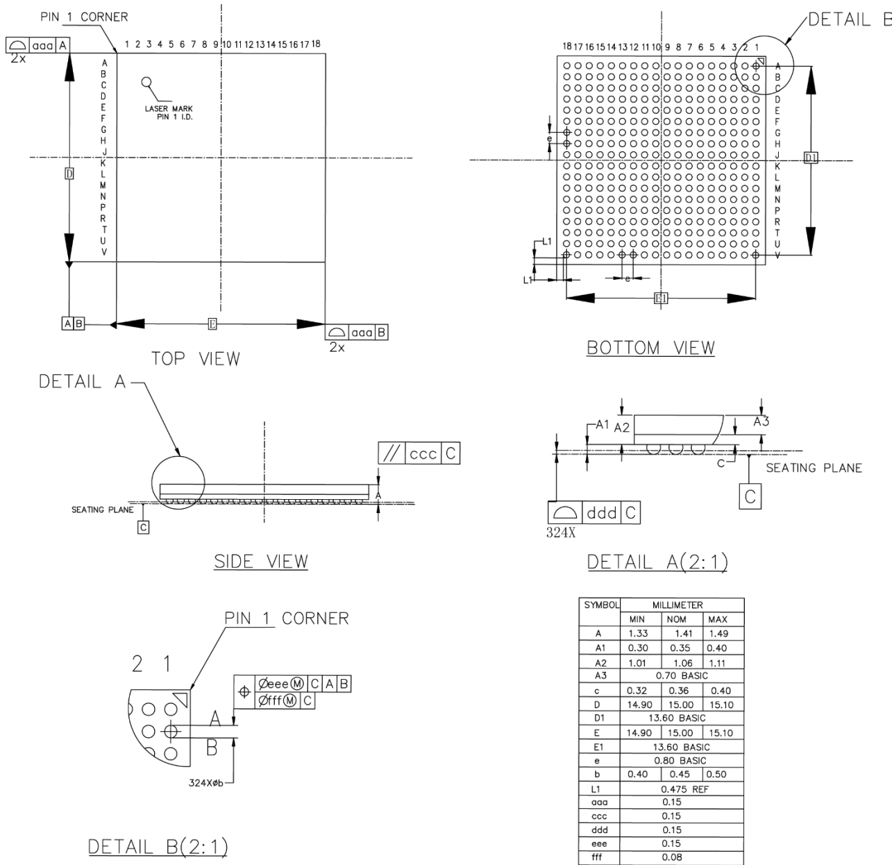
图 4-25 封装尺寸 UG324A (GW5AT-60)
