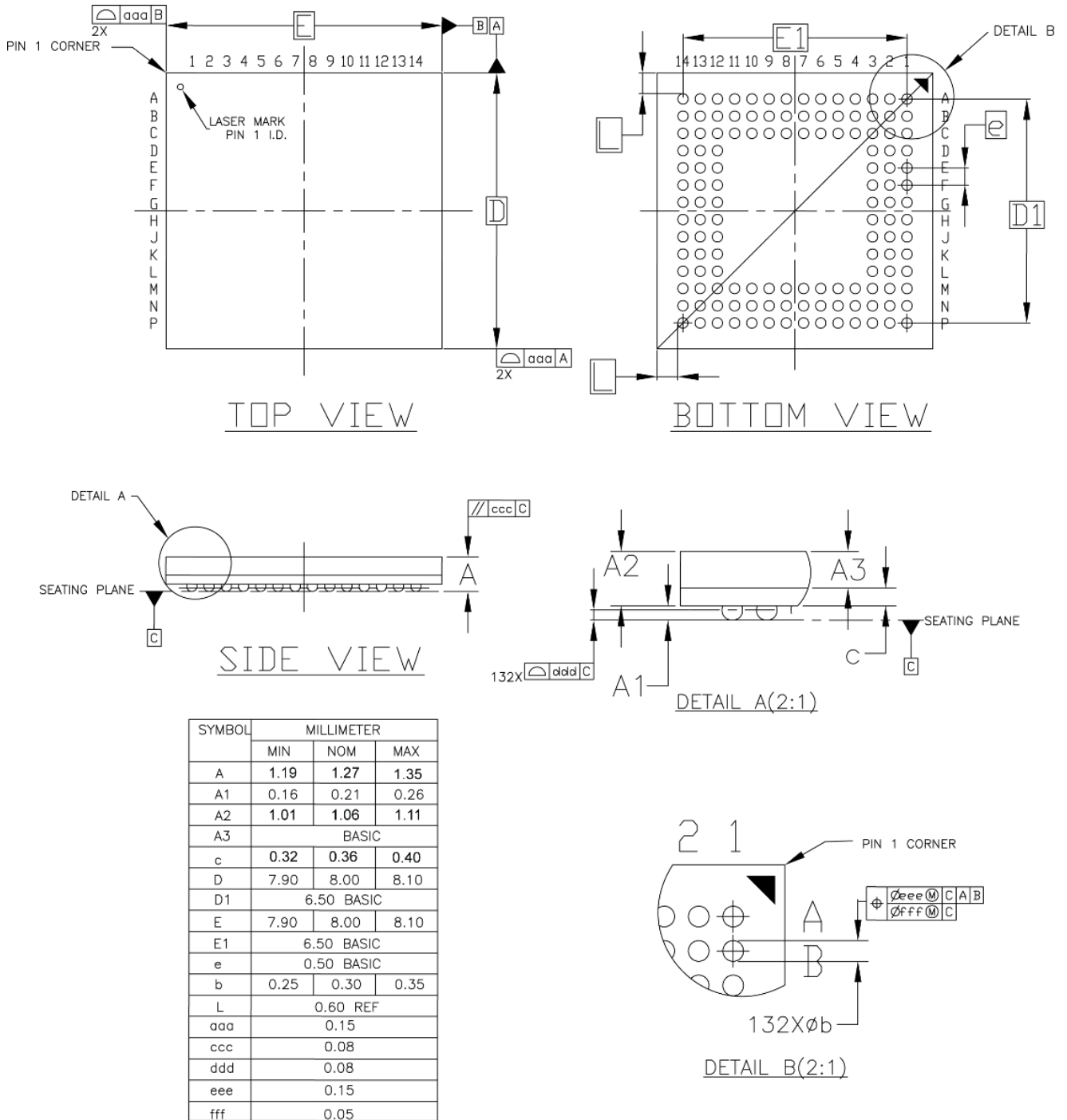
图 4-7 封装尺寸 MG132 (GW5AT-15)
