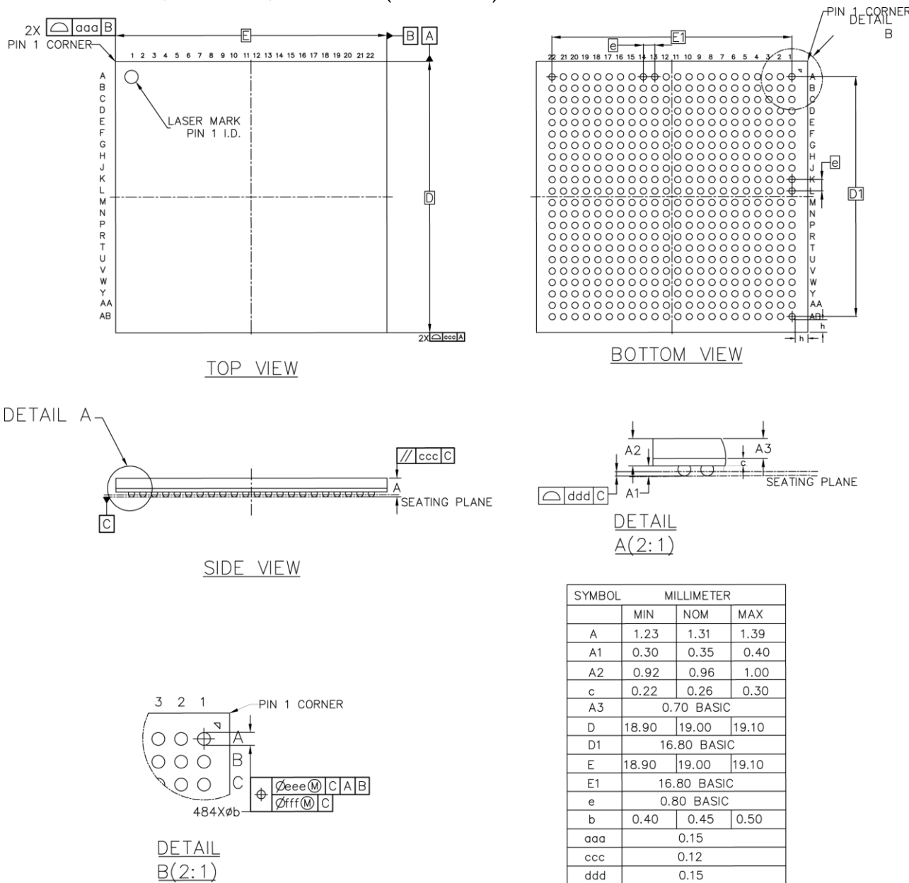
图 4-31 封装尺寸 UG484 (GW5AT-75)
