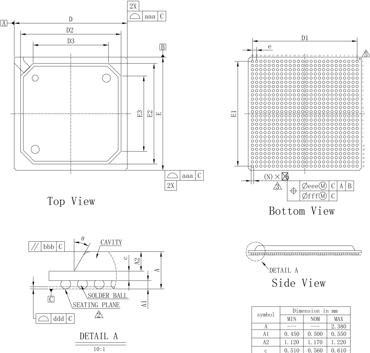
图 4-17 封装尺寸 PG676A (GW5AT-138)
