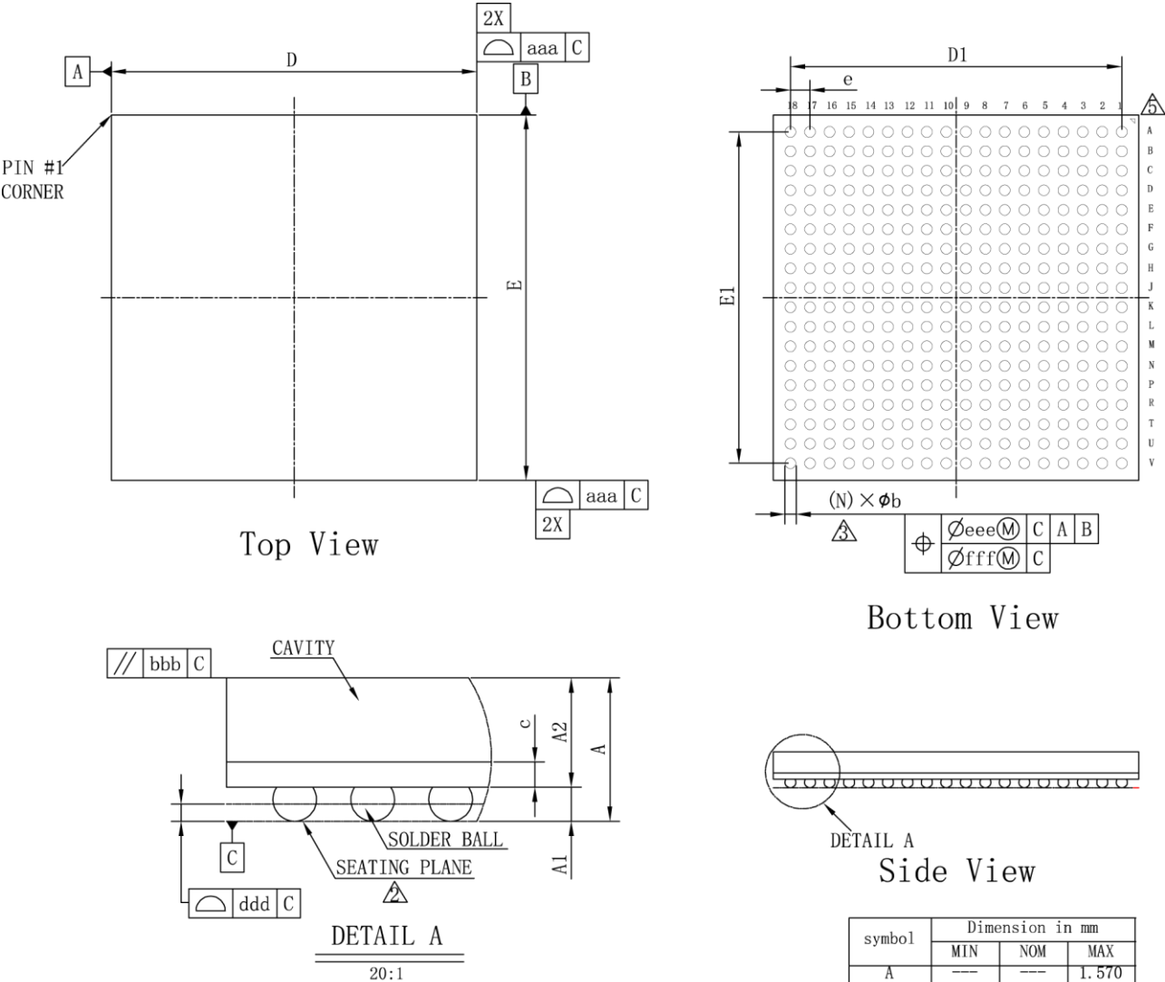
图 4-29 封装尺寸 UG324S (GW5AT-60)
