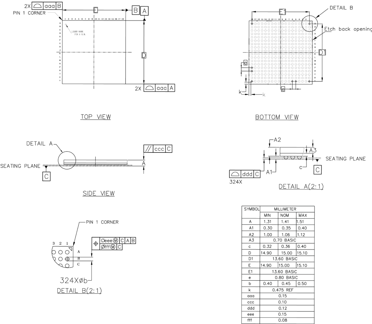
图 4-27 封装尺寸 UG324A (GW5AT-138)
