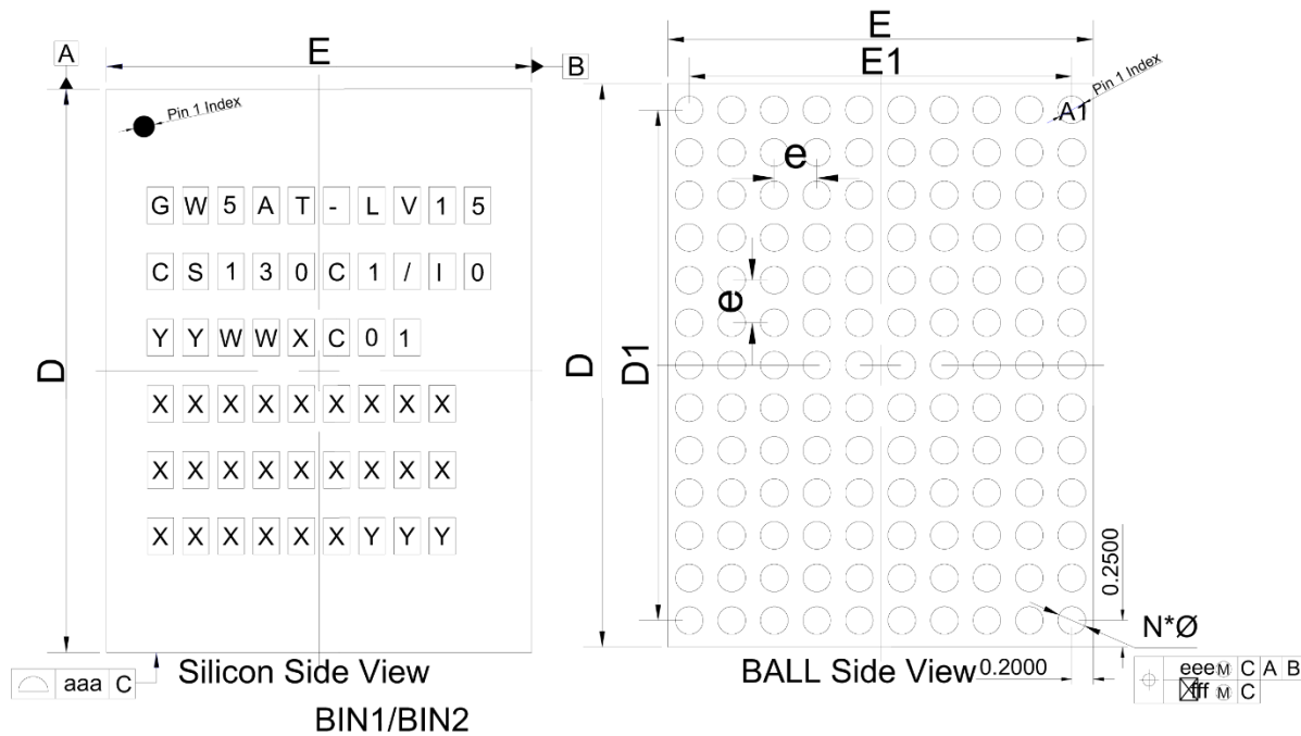
图 4-1 封装尺寸 CS130 (GW5AT-15)
