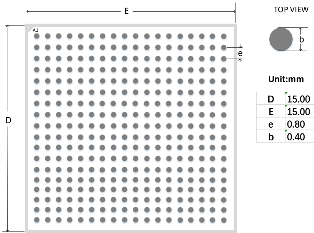
图 4-26 推荐 PCB Layout UG324A (GW5AT-60)
