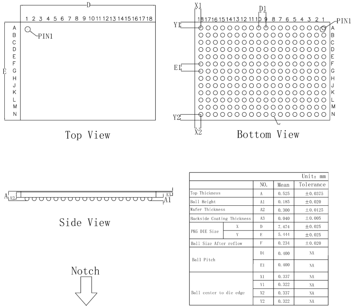
图 4-3 封装尺寸 CS234 (GW5AT-60)
