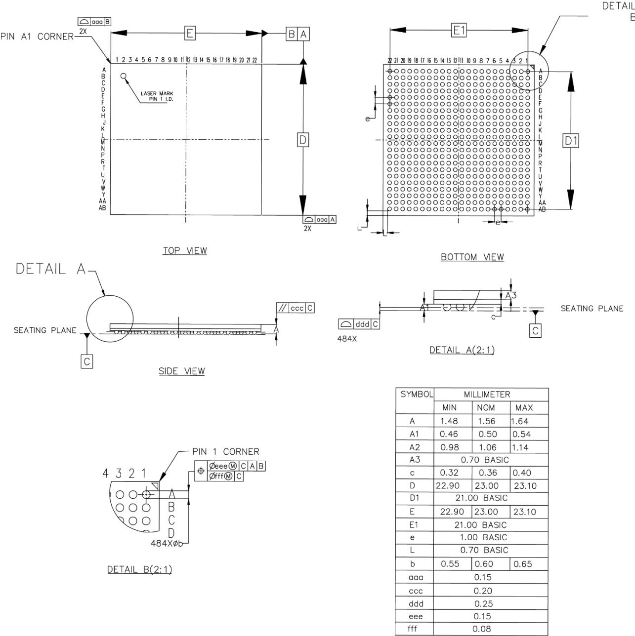
图 4-15 封装尺寸 PG484F (GW5AT-138)
