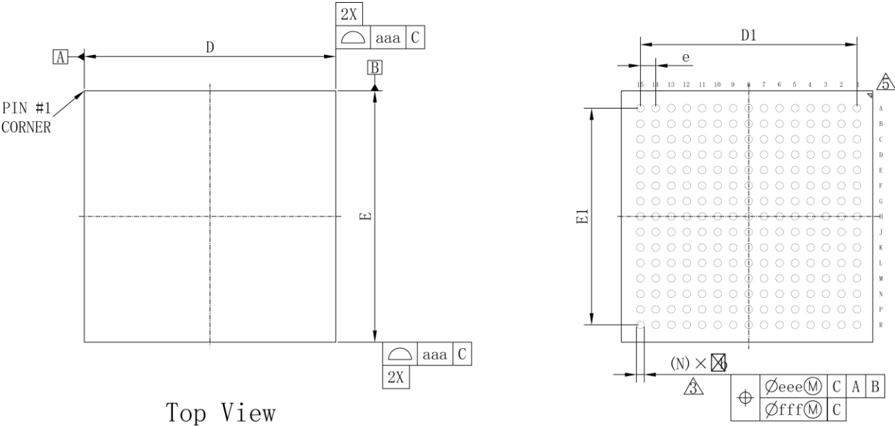
图 4-19 封装尺寸 UG225 (GW5AT-60)
