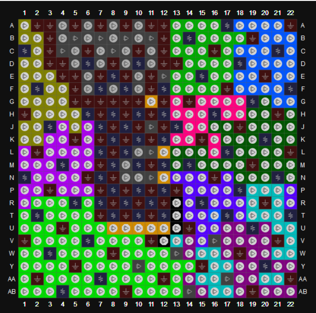
图 3-5 GW5AT-60 器件 PG484A 封装管脚分布示意图（顶视图）
