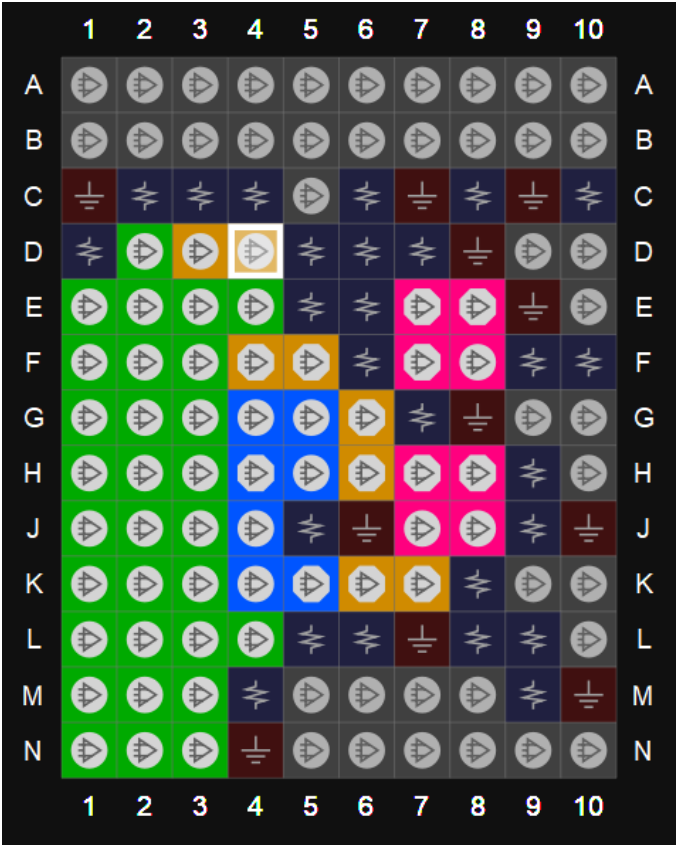
图 3-3 GW5AT-15 器件 CS130F 封装管脚分布示意图（顶视图）
