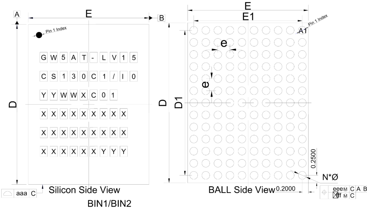
图 4-1 封装尺寸 CS130/CS130F (GW5AT-15)
