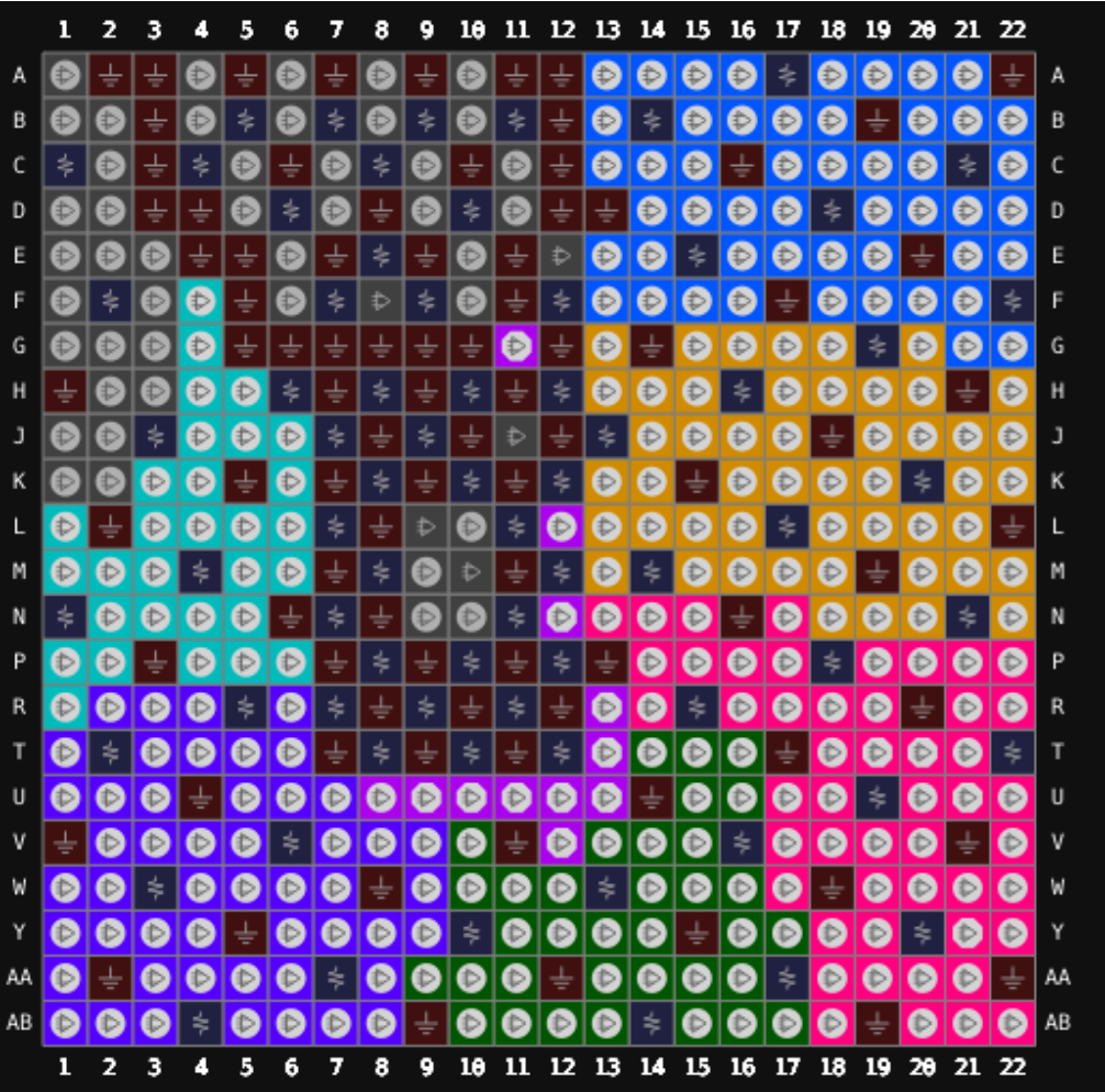
图 3-13 GW5AT-138 器件 PG484 封装管脚分布示意图（顶视图）
