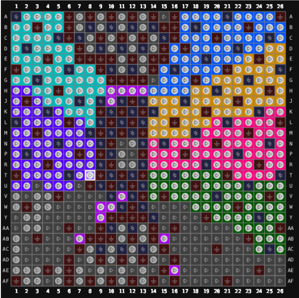
图 3-16 GW5AT-138 器件 PG676A 封装管脚分布示意图（顶视图）
