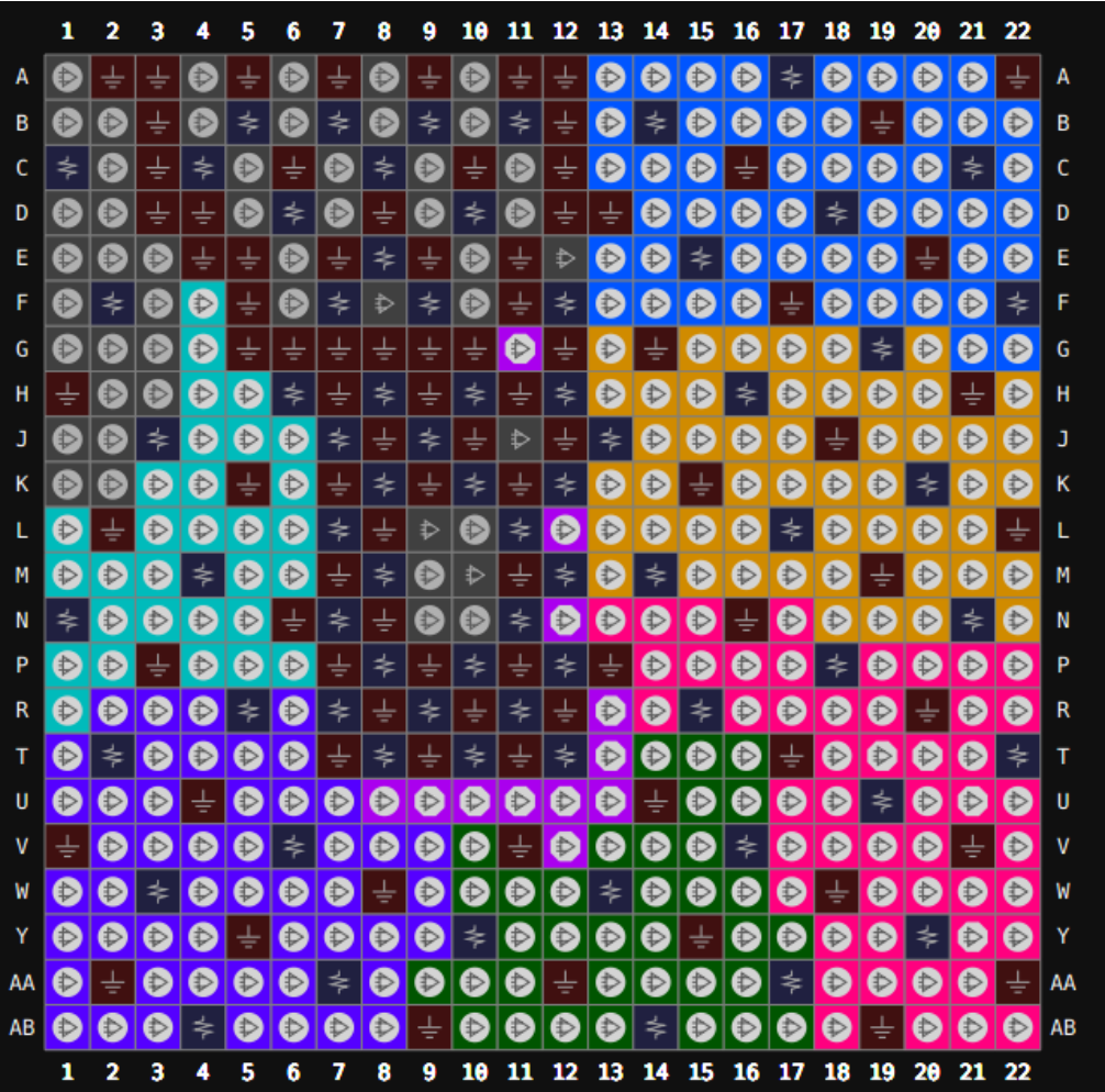
图 3-15 GW5AT-138 器件 PG484F 封装管脚分布示意图（顶视图）
