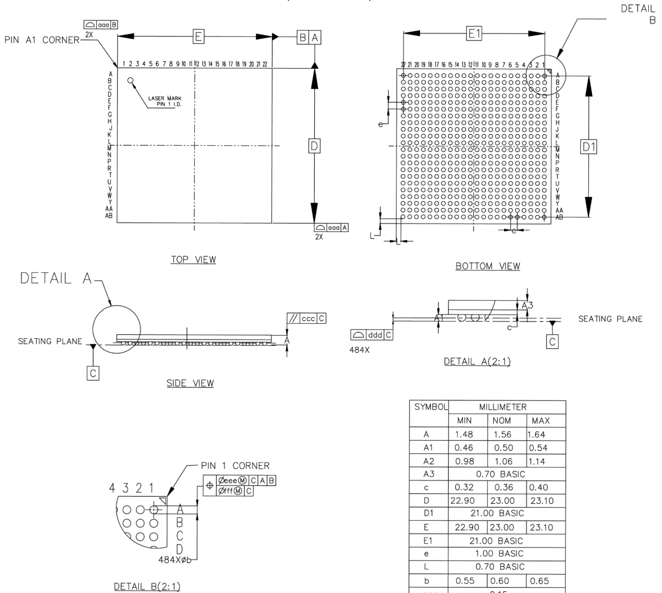
图 4-15 封装尺寸 PG484F (GW5AT-138)
