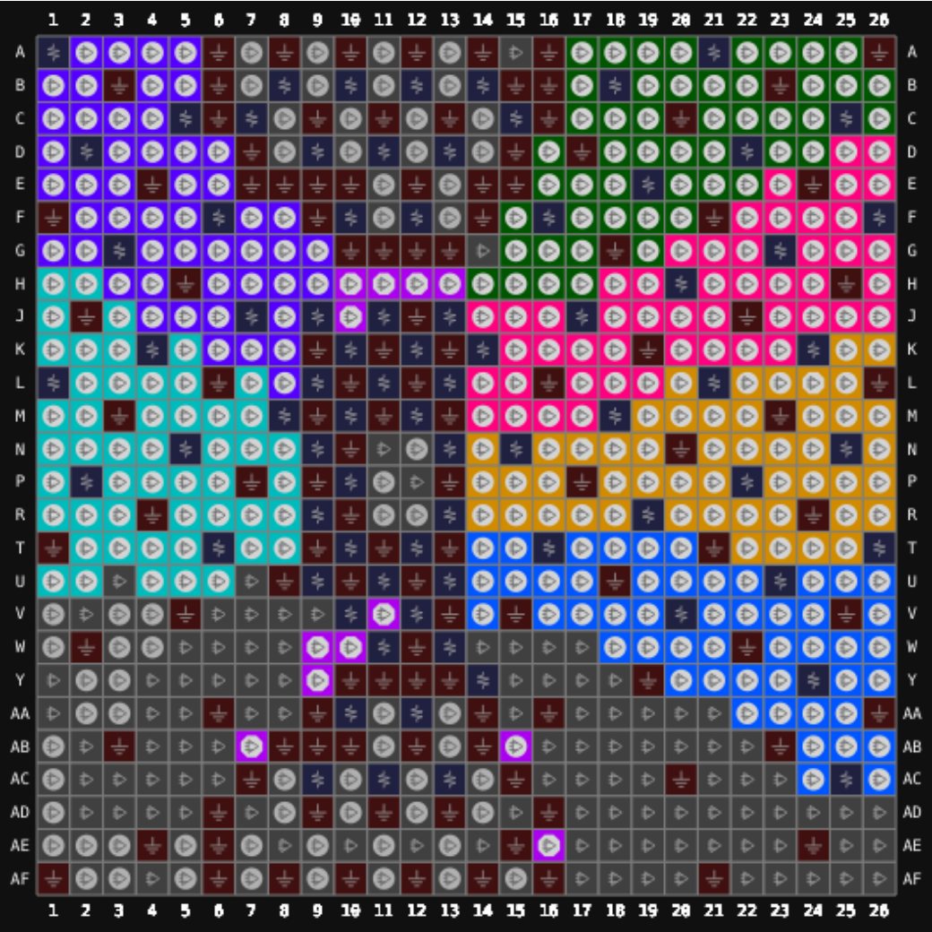
图 3-12 GW5AT-138 器件 FPG676A（Flip Chip）封装管脚分布示意图（顶视图）
