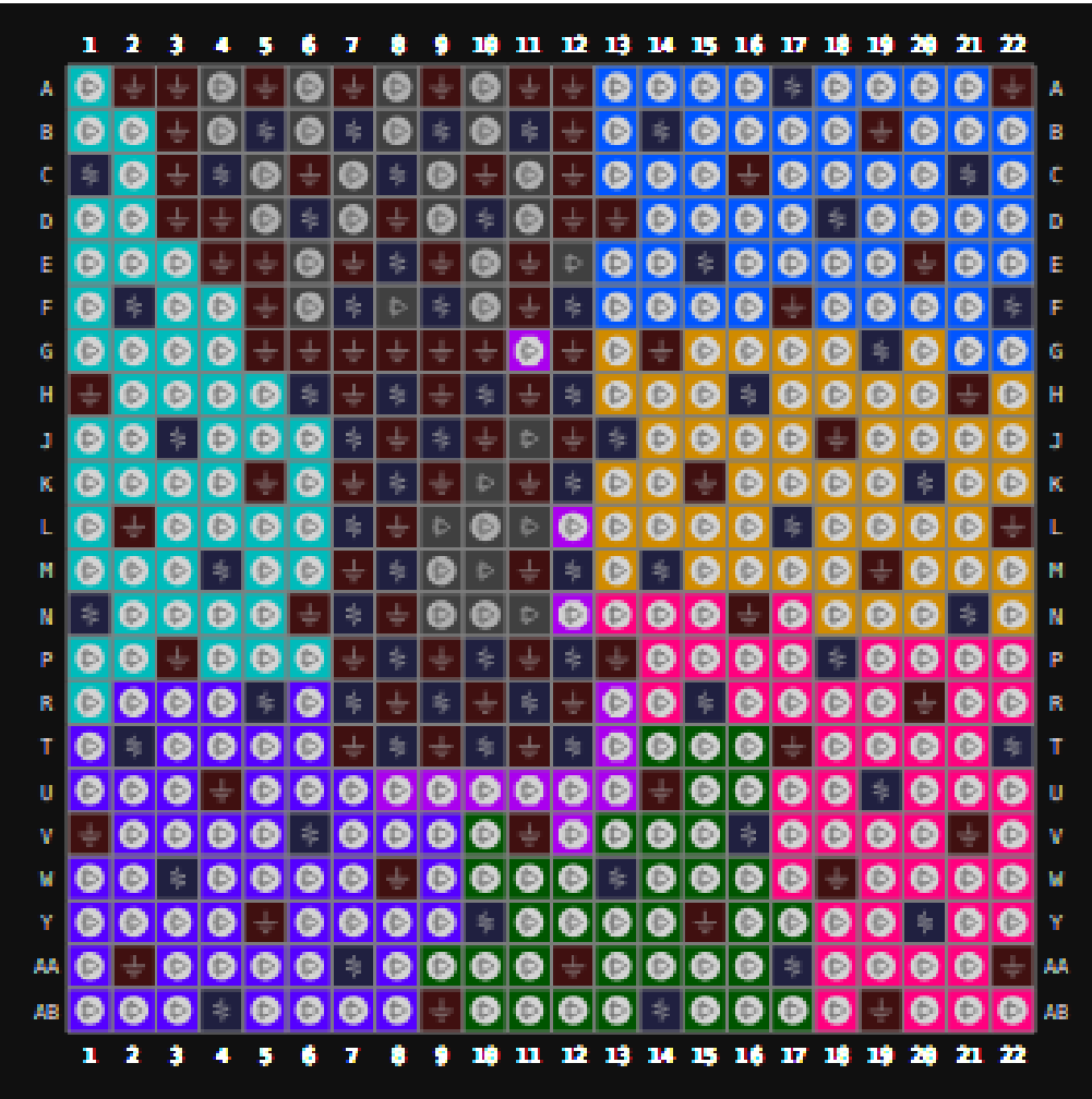
图 3-14 GW5AT-138 器件 PG484A 封装管脚分布示意图（顶视图）
