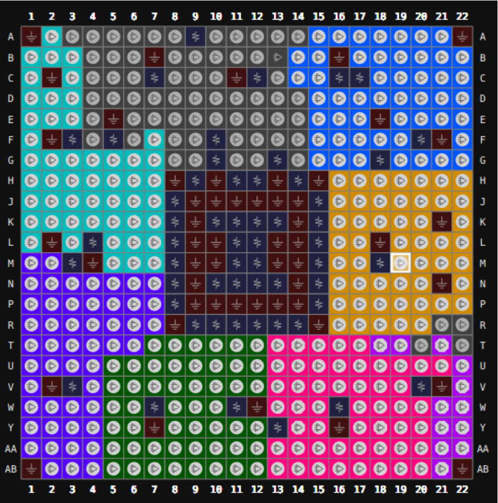
图 3-11 GW5AT-75 器件 UG484 封装管脚分布示意图（顶视图）
