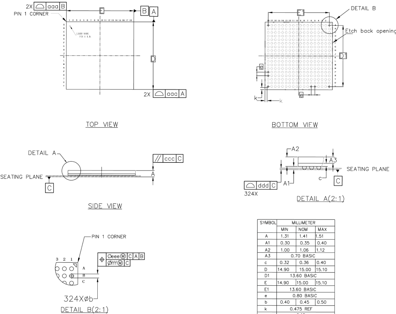
图 4-27 封装尺寸 UG324A (GW5AT-138)
