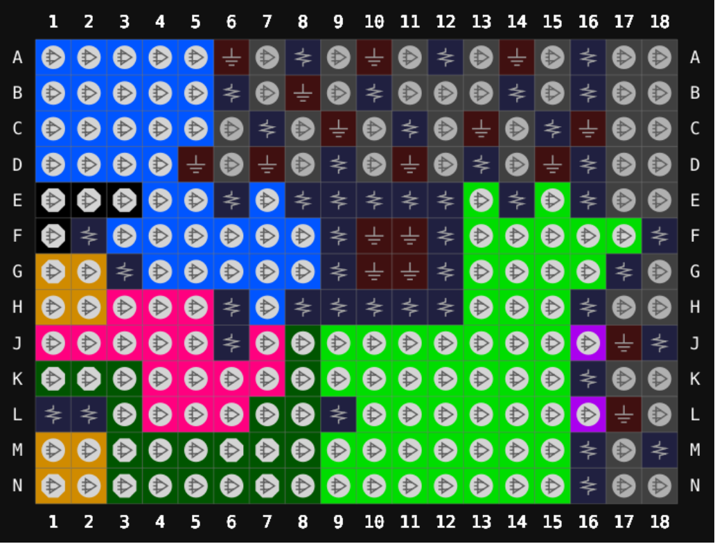
图 3-4 GW5AT-60 器件 CS234 封装管脚分布示意图（顶视图）
