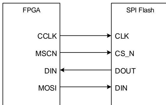
图 4-2 MSPIx1 配置模式连接示意图
