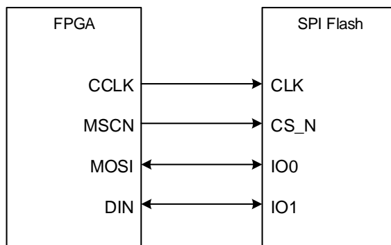
图 4-3 MSPIx2 配置模式连接示意图
