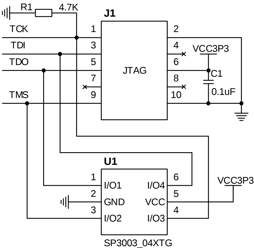
图 4-1 JTAG 配置模式连接示意图
