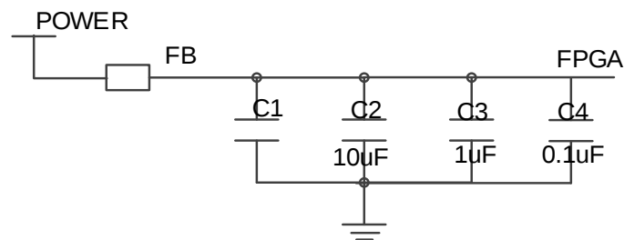
图 2-1 隔离滤波
