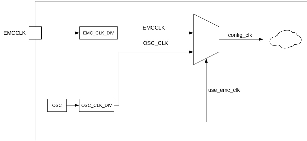
图 3-2 EMCCLK 与 CCLK 图解
