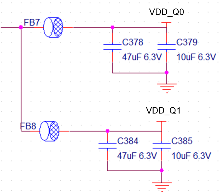
图 2-2 磁珠隔离
