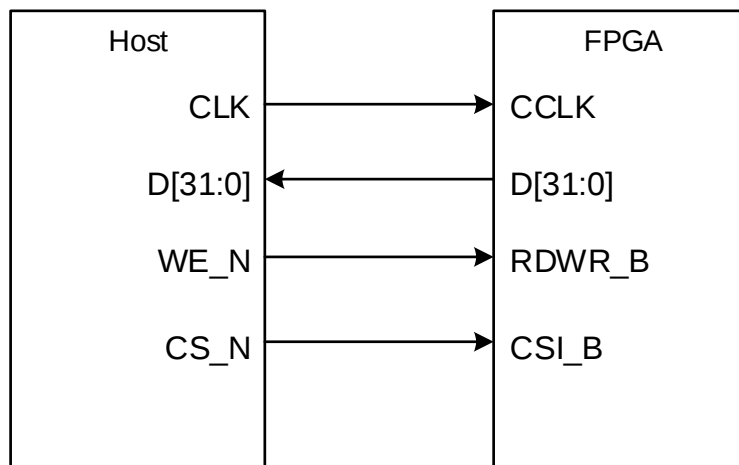
图 4-7 CPU 配置模式连接示意图
