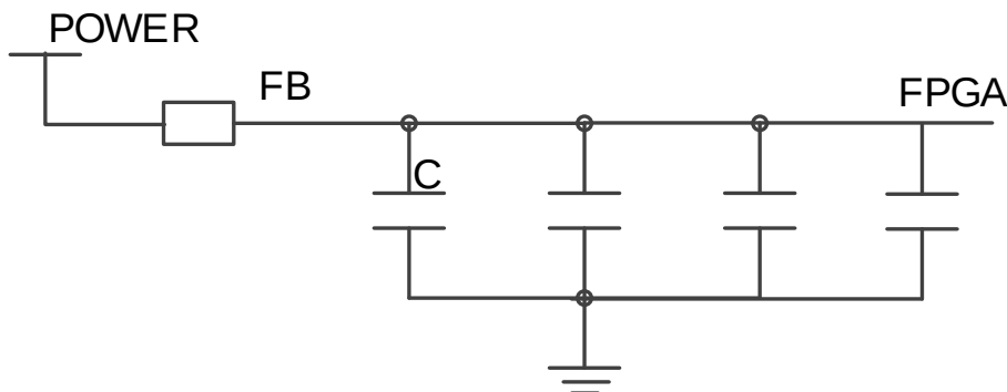
图 2-1 隔离滤波
