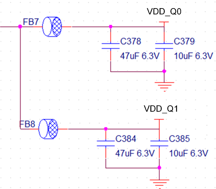
图 2-2 磁珠隔离
