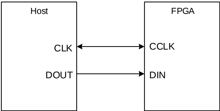
图 4-8 SERIAL 配置模式连接示意图
