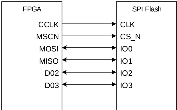
图 4-4 MSPIx4 配置模式连接示意图
