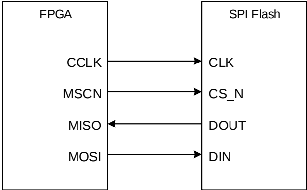
图 4-2 MSPIx1 配置模式连接示意图
