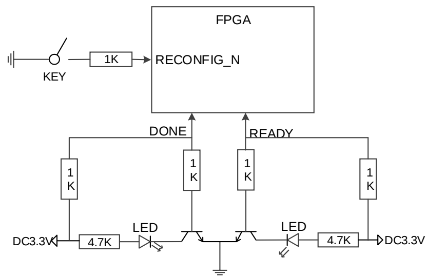
图 3-1 RECONFIG_N, READY, DONE 原理图参考电路
