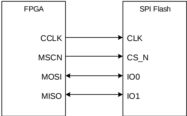
图 4-3 MSPIx2 配置模式连接示意图
