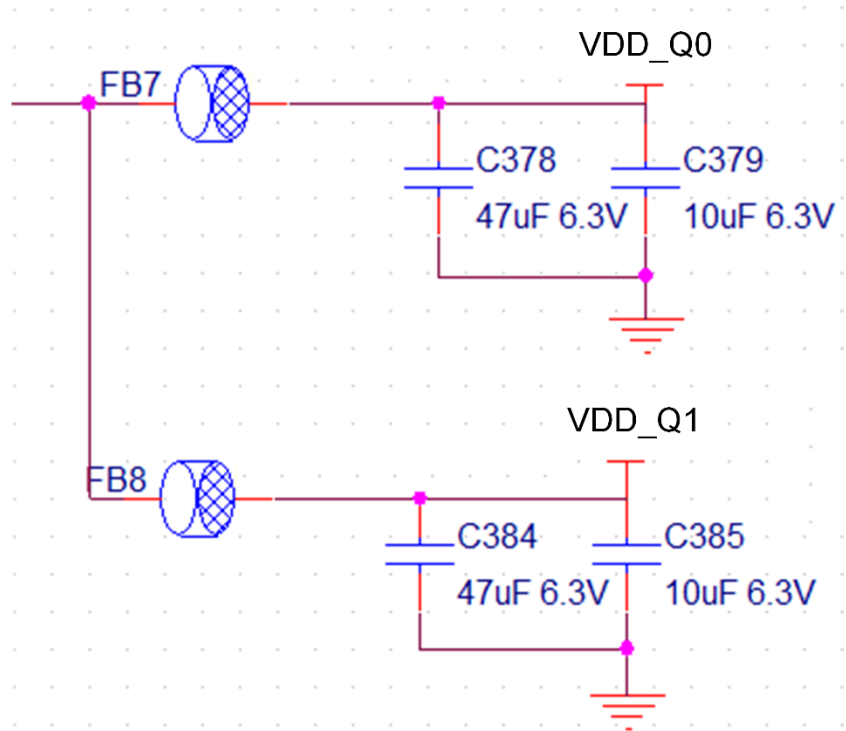
图 2-2 磁珠隔离
