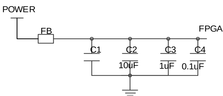
图 2-1 隔离滤波
