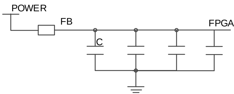
图 2-1 隔离滤波
